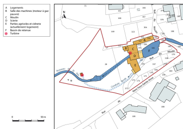
Plan-masse et de situation. Extrait du plan cadastral, 2015, section A. Dess. Mathias Papigny IVR43_20162500944NUDA
