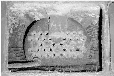
Chaudière de la machine à vapeur : intérieur. Phot. Laurent Poupard IVR43_19913901016Z
