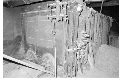
Chaudière de la machine à vapeur. Phot. Laurent Poupard IVR43_19913901014Z
