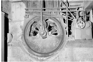
Système d'entraînement du châssis de scie vertical. Phot. Laurent Poupard IVR43_19913900996Z
