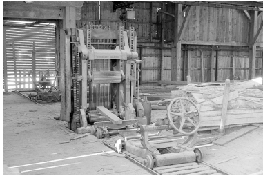
Châssis de scie vertical Socolest. Phot. Laurent Poupard IVR43_19913900995Z
