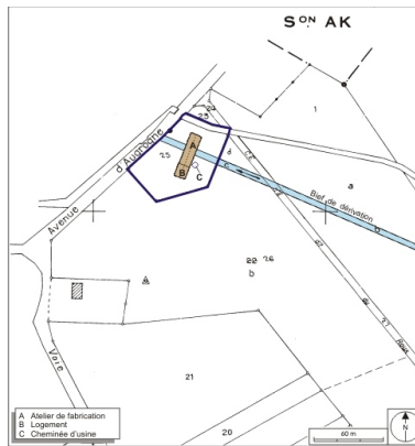
Plan-masse et de situation. Extrait du plan cadastral, 2008, section ZI, 1:2000. Source : Direction générale des Finances Publiques - Cadastre ; mise à jour : 2008. Dess. André Céréza IVR43_20087000199NUDA
