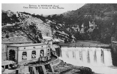
Environs de Moirans (Jura). Usine Electrique et barrage du Saut Mortier. Phot. Yves Sancey IVR43_19883900431X
