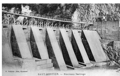
Saut-Mortier. - Nouveau Barrage. Phot. Yves Sancey, Phot. F. Vialatte IVR43_19883900429X
