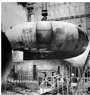
Bâche métallique CAFL en cours d'acheminement par le pont roulant et avant sa mise en place sur sa murette support.
