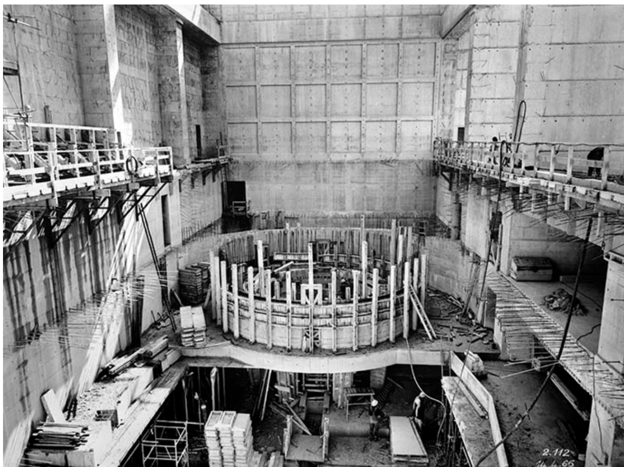
Intérieur de l'usine en cours de construction.
