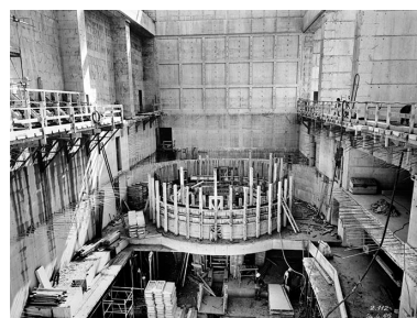
Intérieur de l'usine en cours de construction. Phot. Jérôme Mongreville, Autr. H. Baranger et Cie IVR43_19913900325X
