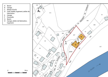
Plan-masse et de situation. Dess. Mathias Papigny IVR43_20162501545NUDA
