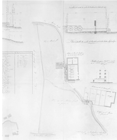
Plan général [...] du canal du moulin de Courtelevant et du battoir hydraulique que se propose d'établir François Marion [...]. Phot. Jérôme Mongreville, Autr. E. Bogard IVR43_20019000250X
