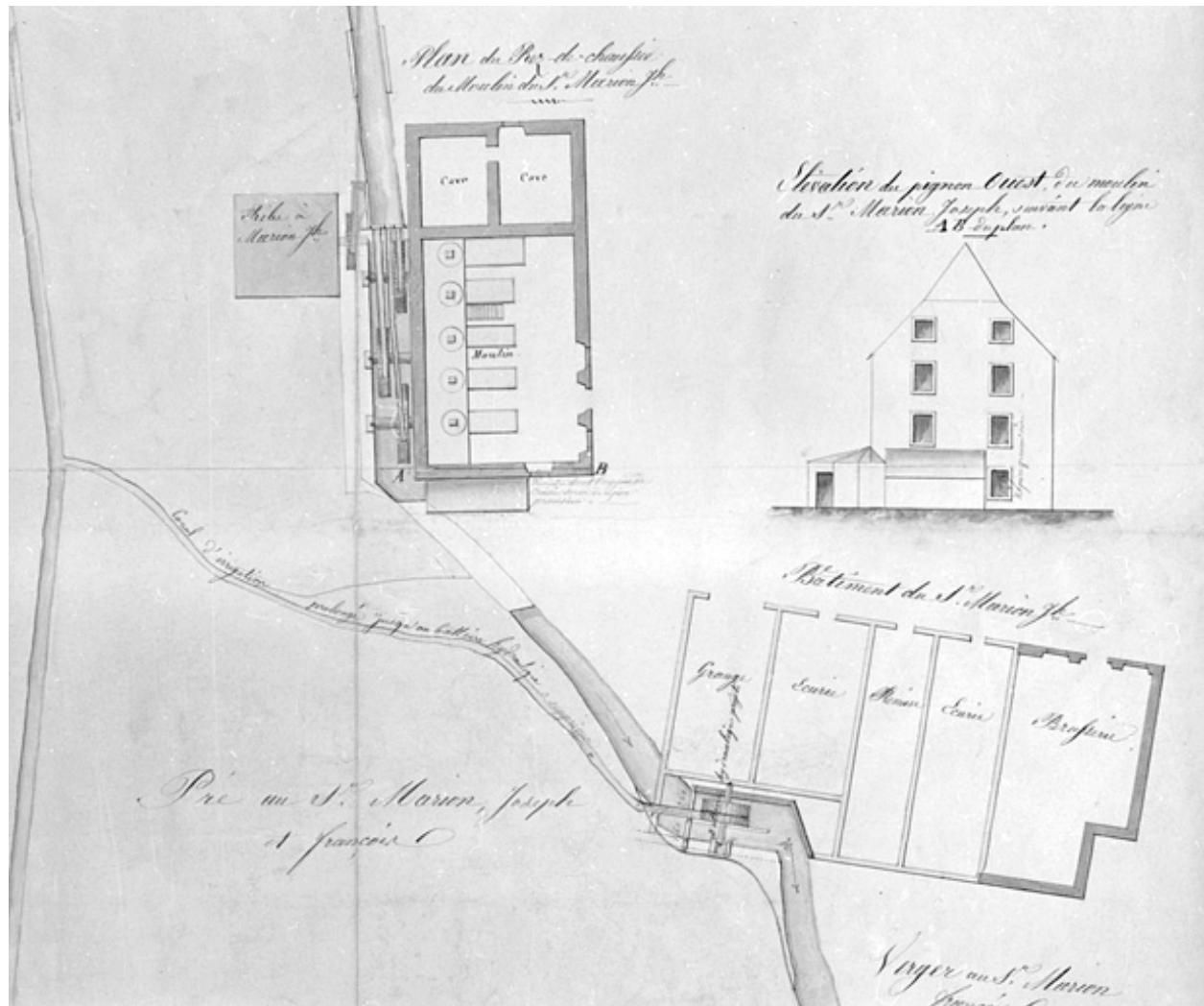
Plan général [...] du canal du moulin de Courtelevant et du battoir hydraulique que se propose d'établir François Marion [détail].
