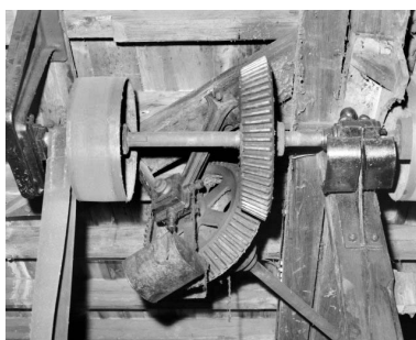
Renvoi de la transmission vers l'atelier de filature (N). Phot. Yves Sancey IVR43_19943901563X
