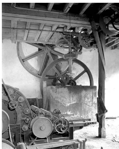
Transmission de la grande roue hydraulique. Phot. Yves Sancey IVR43_19943901562X
