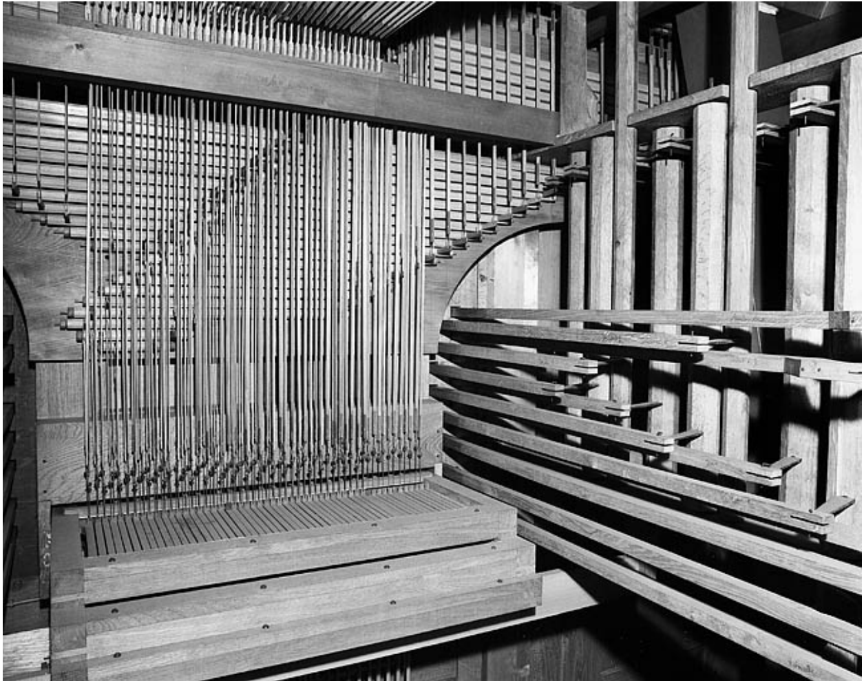
Mécanique vue de trois quarts gauche.
