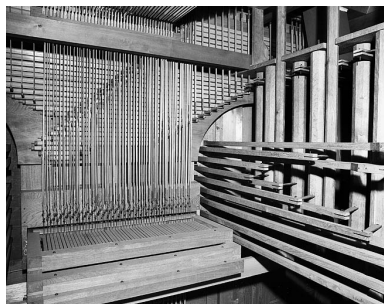
Mécanique vue de trois quarts gauche. Phot. Jérôme Mongreville IVR43_19862500436X
