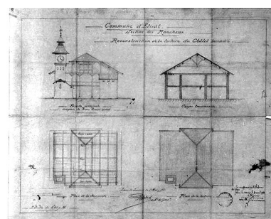
Commune d'Etival [...] [plans, coupe et élévation]. Reconstruction de la toiture du châtelet incendié [plans, coupe et élévation]. Phot. Jérôme Mongreville, Phot. Jules Pelletier IVR43_19963900194X
