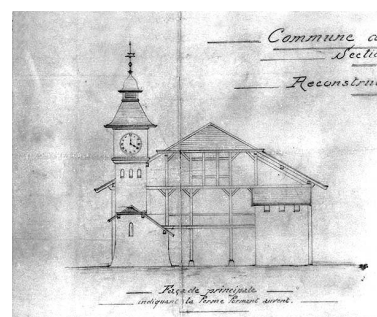
Commune d'Etival [...] [détail : élévation de la façade est]. Reconstruction de la toiture du châtelet incendié [détail : élévation de la façade est]. Phot. Jérôme Mongreville, Phot. Jules Pelletier IVR43_19963900195X
