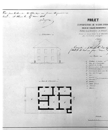
Projet d'appropriation de Maison d'Ecole [...] [plan au rez-de-chaussée et élévation]. Phot. Jérôme Mongreville, Phot. Comoy IVR43_19963900191X
