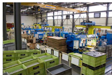
Site récent : un atelier d'injection plastique. Phot. Yves Sancey
