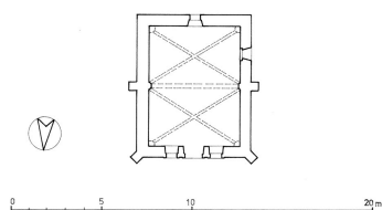
Plan. Dess. Alain Morelière IVR26_20122100522A4YY
