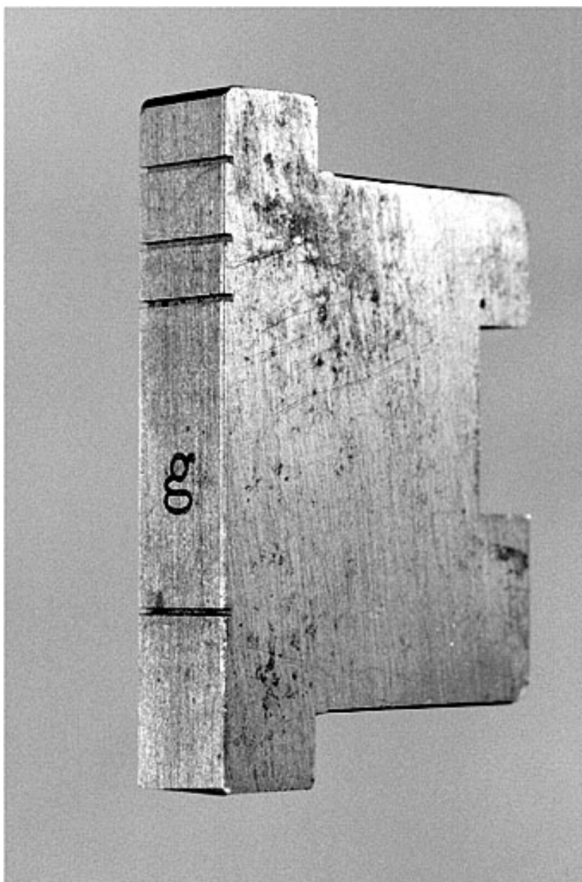
Matrice de caractère (face supérieure).
