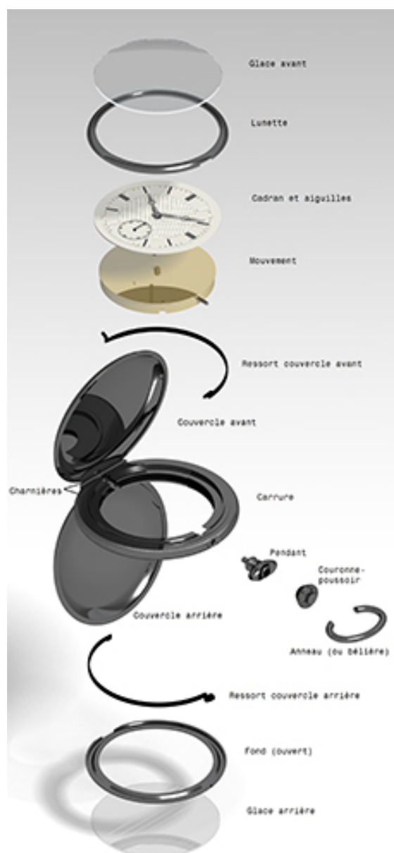
Montre de gousset : présentation éclatée de l'habillage.
