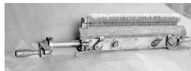
Porte-pierres d'un appareil à cylindre. Les pierres étaient collées sur les batonnets métalliques. Phot. Laurent Poupard IVR43_19913901040Z
