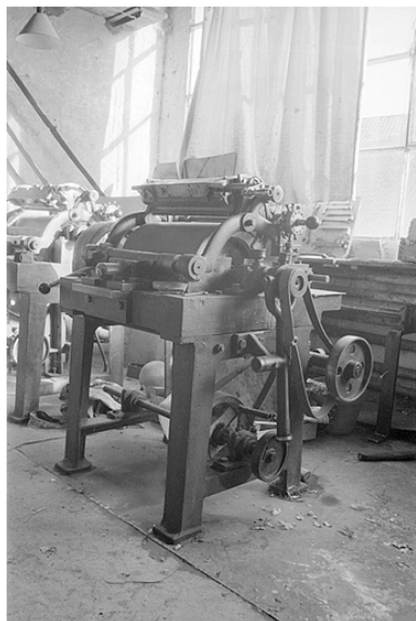
Appareil à cylindre. Porte-pierres baissé. Phot. Laurent Poupard IVR43_19913901038Z
