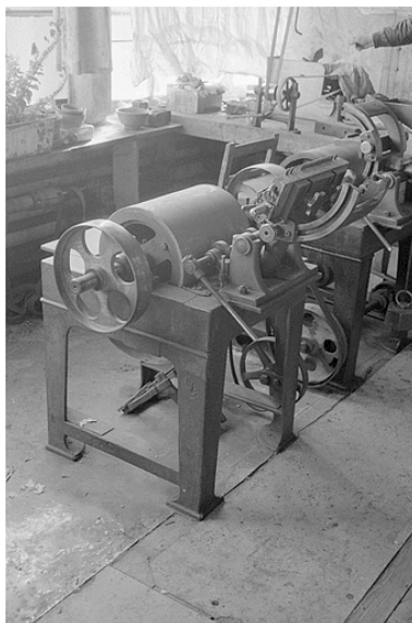
Appareil à cylindre. Porte-pierres levé. Phot. Laurent Poupard IVR43_19913901039Z
