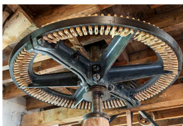
Roue métallique engrenée de dents (alluchons) en bois, appelée rouet. Phot. Jérôme Mongreville IVR43_20162500277NUC4A
