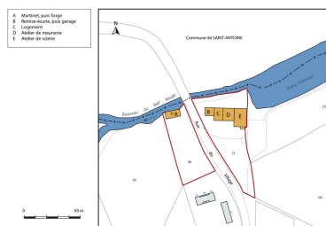
Plan-masse et de situation. Extrait du plan cadastral, 2015, section AE. Dess. Mathias Papigny IVR43_20162500933NUDA
