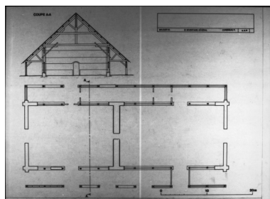
Plan et coupe de la halle à charbon. Relevé graphique, 1988, M. Brugier et F. Corbineau, échelle 1:1250. Phot. Yves Sancey IVR43_19937000008X
