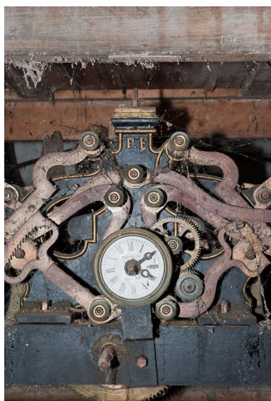
Mécanisme d'horloge : détail. Phot. Pierre-Marie Barbe-Richaud IVR26_20112100624NUC2A
