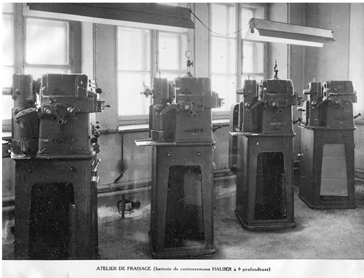
Atelier de fraisage (batterie de contourneuses Hauser à 9 profondeurs), vers 1950.
