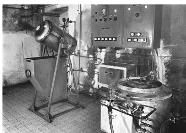
USINE DE TRAITEMENT THERMIQUE (trempe blanche et revenu en atmosphère contrôlée)
