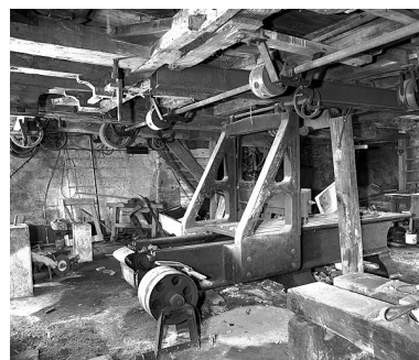
Partie arrière : poulies et engrenages d'entraînement de la table. En côté de l'entretoise, manivelle de réglage en hauteur de la traverse porte-outil. Phot. Yves Sancey IVR43_19943901360X
