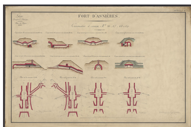
Fort d'Asnières. Casemates à canons n° 66, 67, 68 et 69. 1885. Phot. Petot Frédéric, Autr. auteur inconnu
