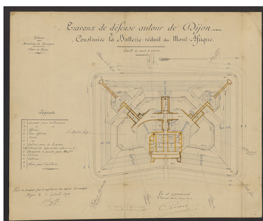
Travaux de défense autour de Dijon - Construire la batterie réduit du Mont-Afrique. 1878. Phot. Petot Frédéric, Autr. auteur inconnu IVR26_20252100180NUC4A
