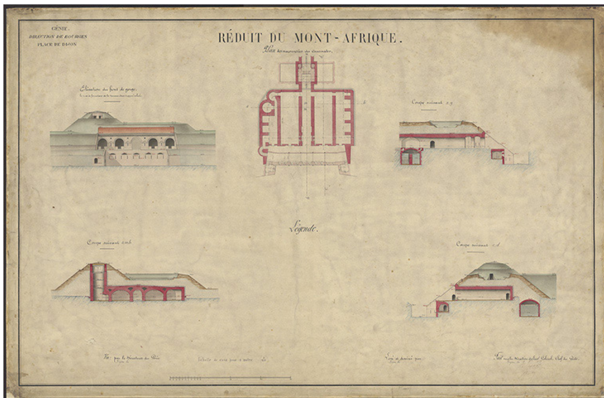
Réduit du Mont-Afrique. Plan des maçonneries des casemates. 1885.
