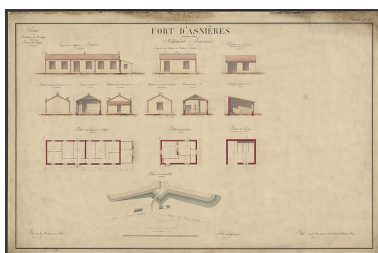
Fort d'Asnières. Bâtiments annexes. 1885. Phot. Petot Frédéric, Autr. auteur inconnu
