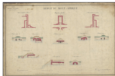
Réduit du Mont-Afrique. Plan des abris, latrines, magasin à poudre et cuisine. 1885. Phot. Petot Frédéric, Autr. auteur inconnu IVR26_20252100176NUC4A
