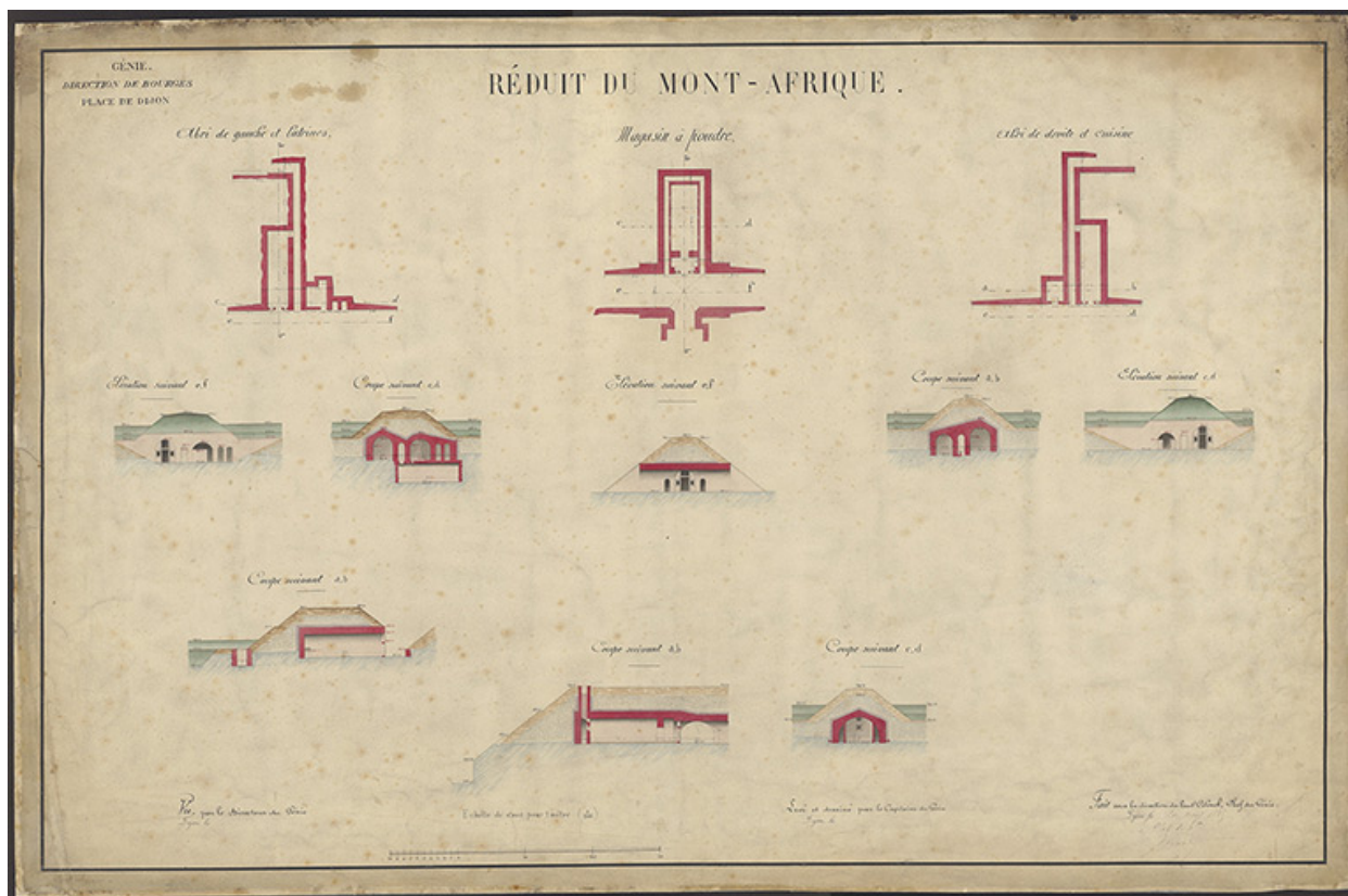
Réduit du Mont-Afrique. Plan des abris, latrines, magasin à poudre et cuisine. 1885.
