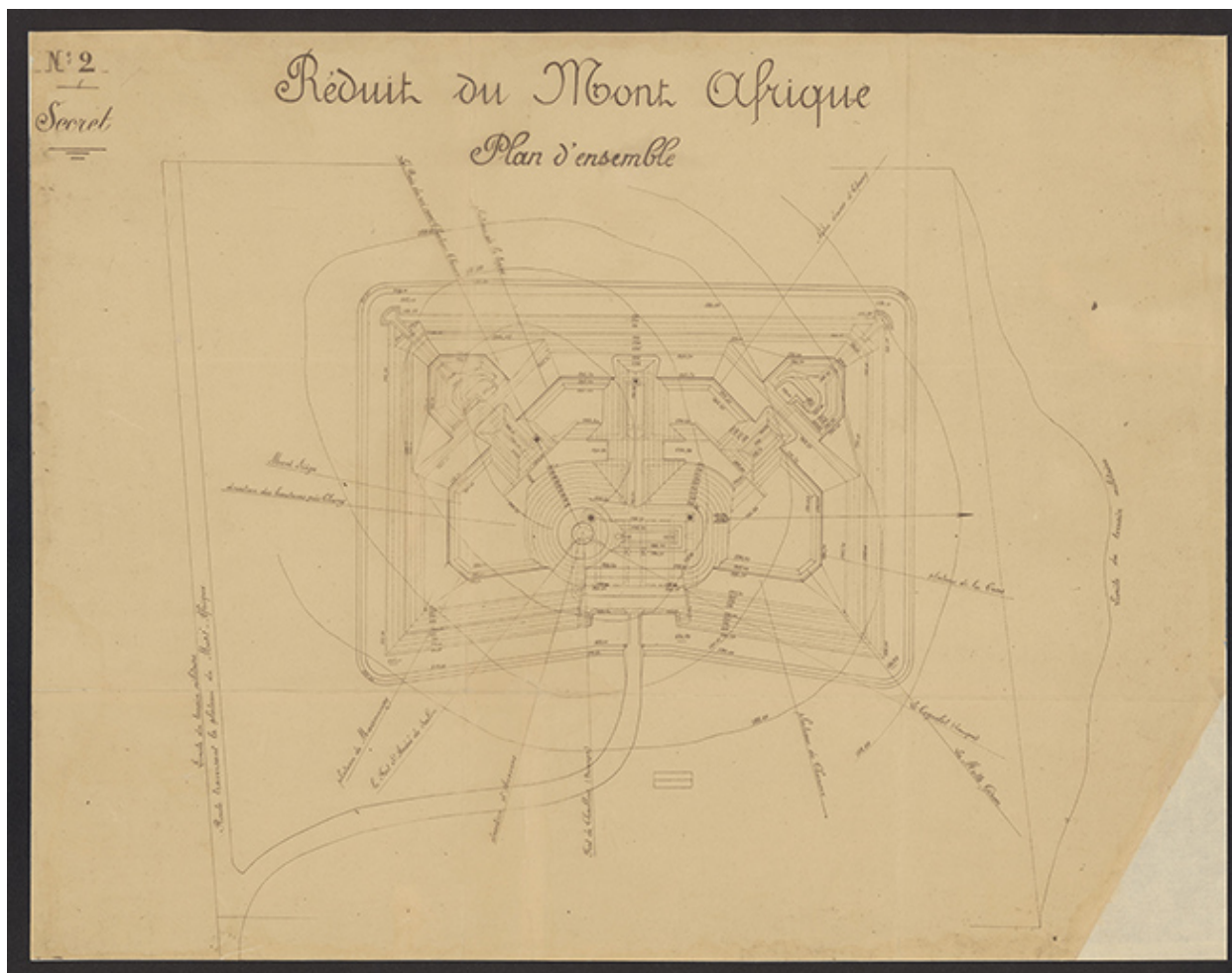
Réduit du Mont-Afrique. Plan d'ensemble. S.d.
