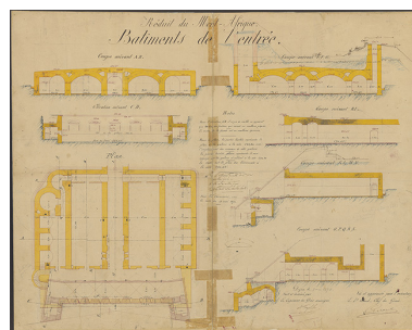
Réduit du Mont-Afrique. Bâtiments de l'entrée. 1878. Phot. Petot Frédéric, Autr. auteur inconnu IVR26_20252100178NUC4A
