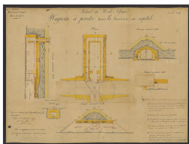
Réduit du Mont-Afrique. Magasin à poudre sous la traverse en capitale. 1877. Phot. Petot Frédéric, Autr. auteur inconnu IVR26_20252100182NUC4A
