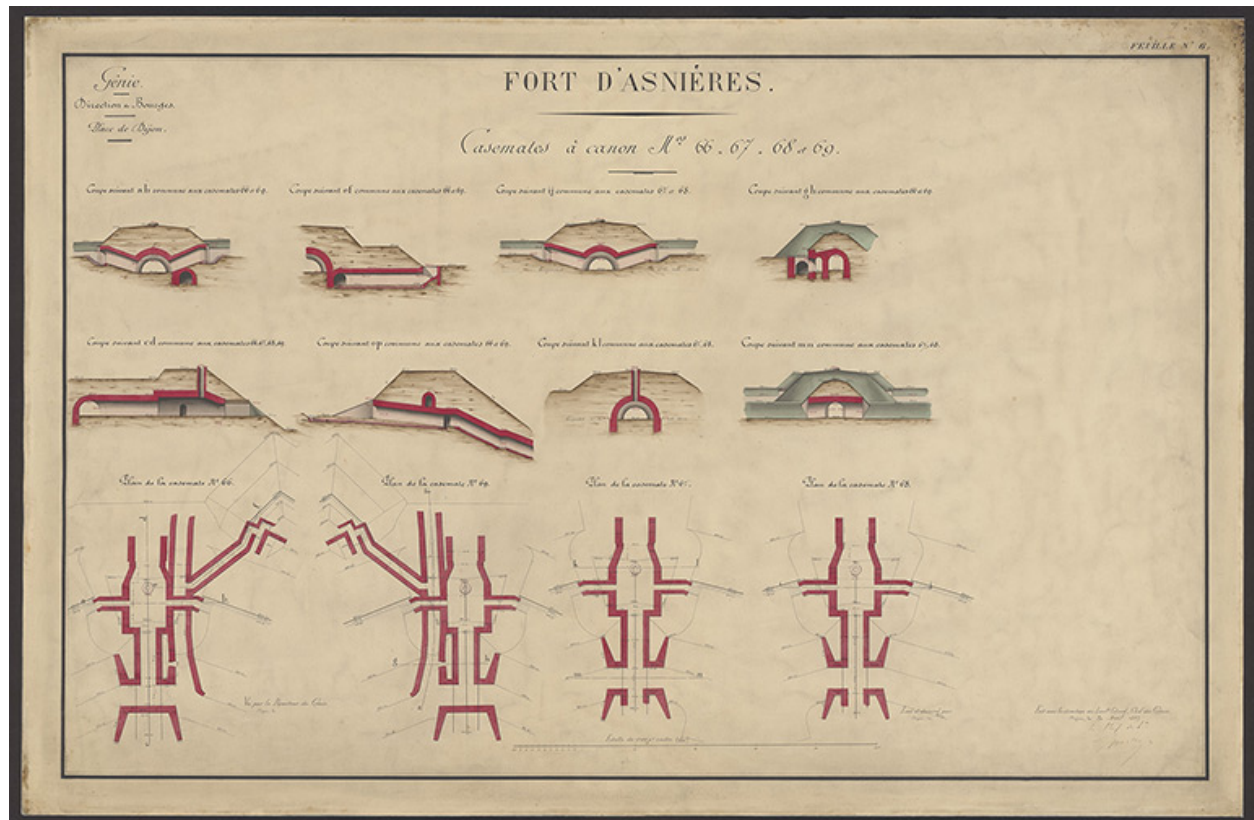
Fort d'Asnières. Casemates à canons n° 66, 67, 68 et 69. 1885.
