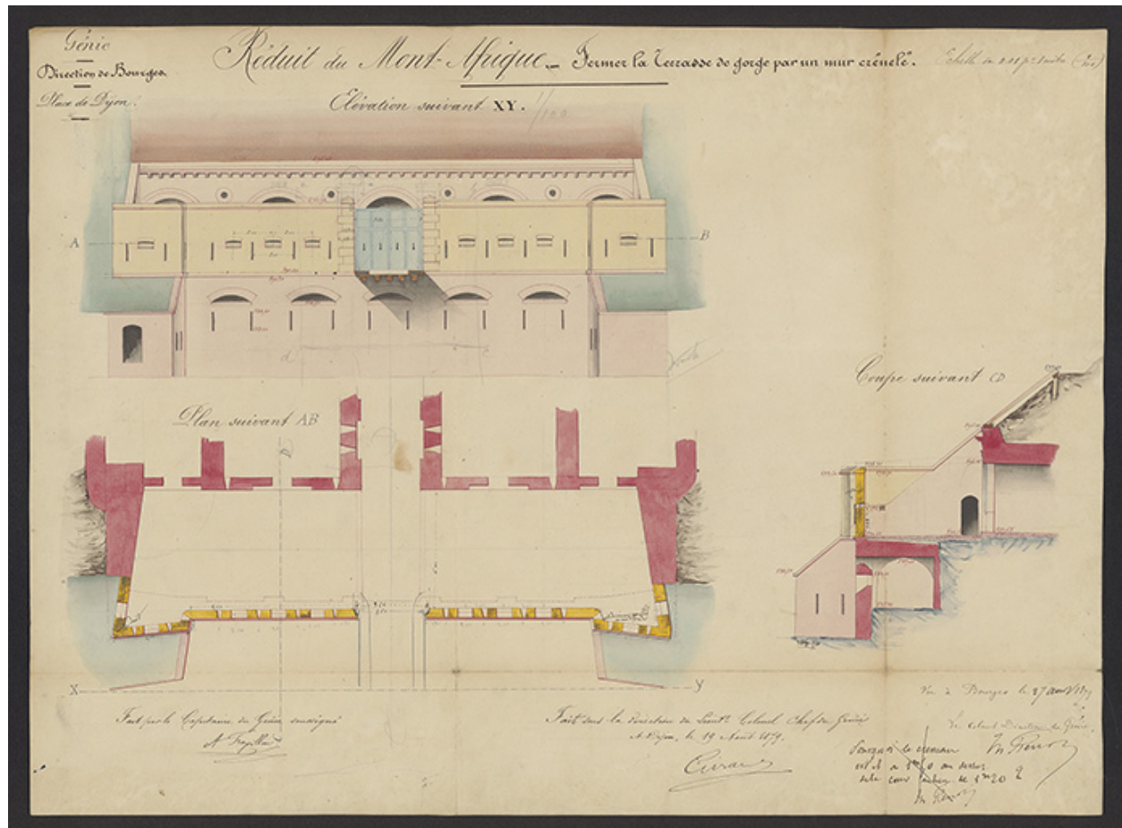
Rêduit du Mont-Afrique. [la terrasse de gorge et son mur crénelé]. 1879.
