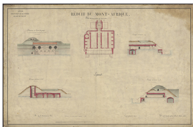
Réduit du Mont-Afrique. Plan des maçonneries des casemates. 1885. Phot. Petot Frédéric, Autr. auteur inconnu IVR26_20252100175NUC4A
