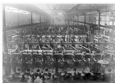
Intérieur de l'atelier central de l'usine. Phot. Jérôme Mongreville IVR43_19913900946V
