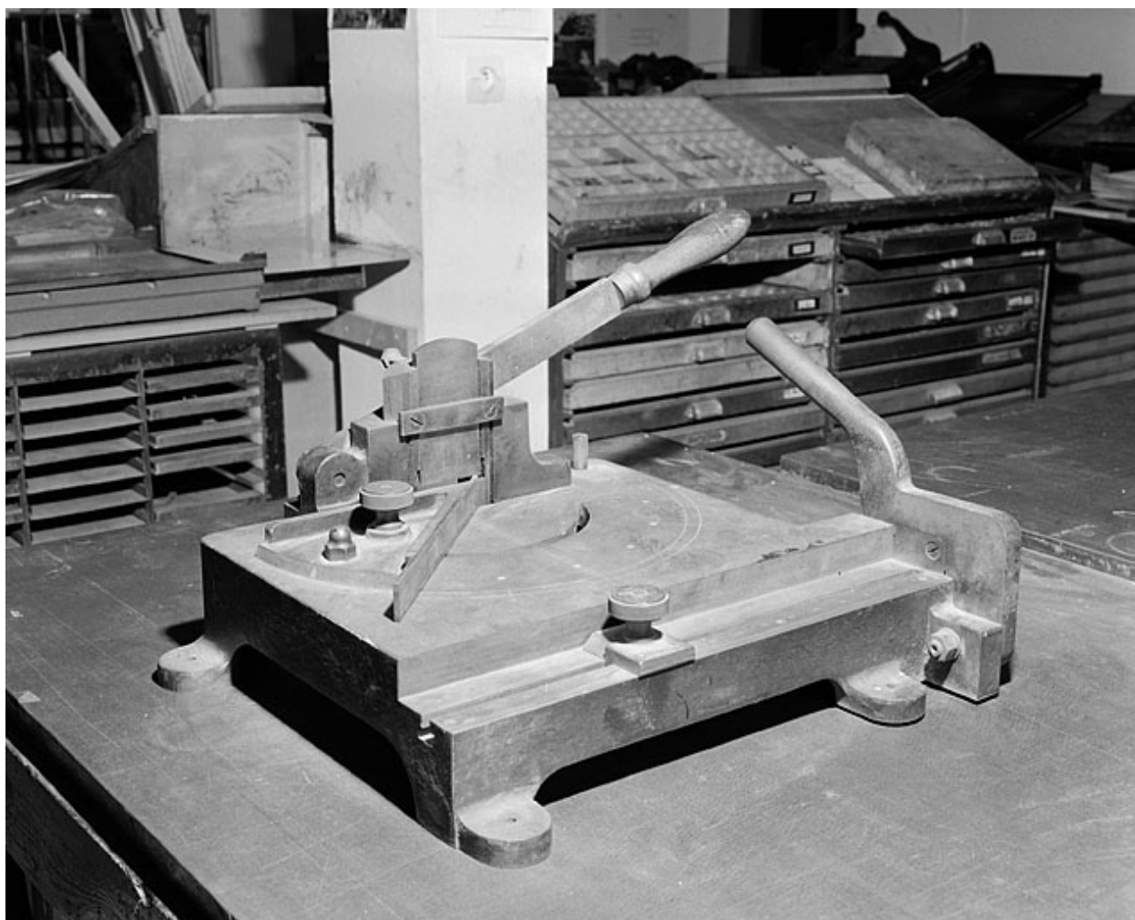
Vue d'ensemble d'un coupleur-biseauteur. "Couteau-rabot" pour les coupes obliques à gauche, "couteau-guillotine" pour les coupes de longueur à droite.
