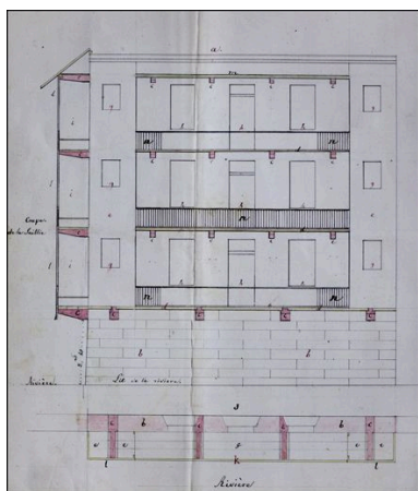
Projet à discuter relatif à la forme qu'il convient d'adopter pour l'établissement de galeries et de latrines dans les façades des maisons de la rue des Promenades du côté de la rivière, 1849. Dessin (plume, lavis), 10 juin 1849, échelle 1:100.
