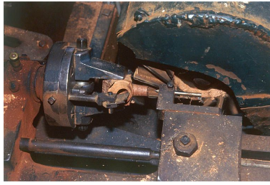
Mandrin gueule de loup et fraise verticale, vue de face en plongée. Phot. Jérôme Mongreville IVR43_20003901055ZA
