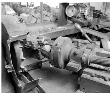
Mandrin gueule de loup et fraise verticale. Phot. Jérôme Mongreville IVR43_20003901056X
