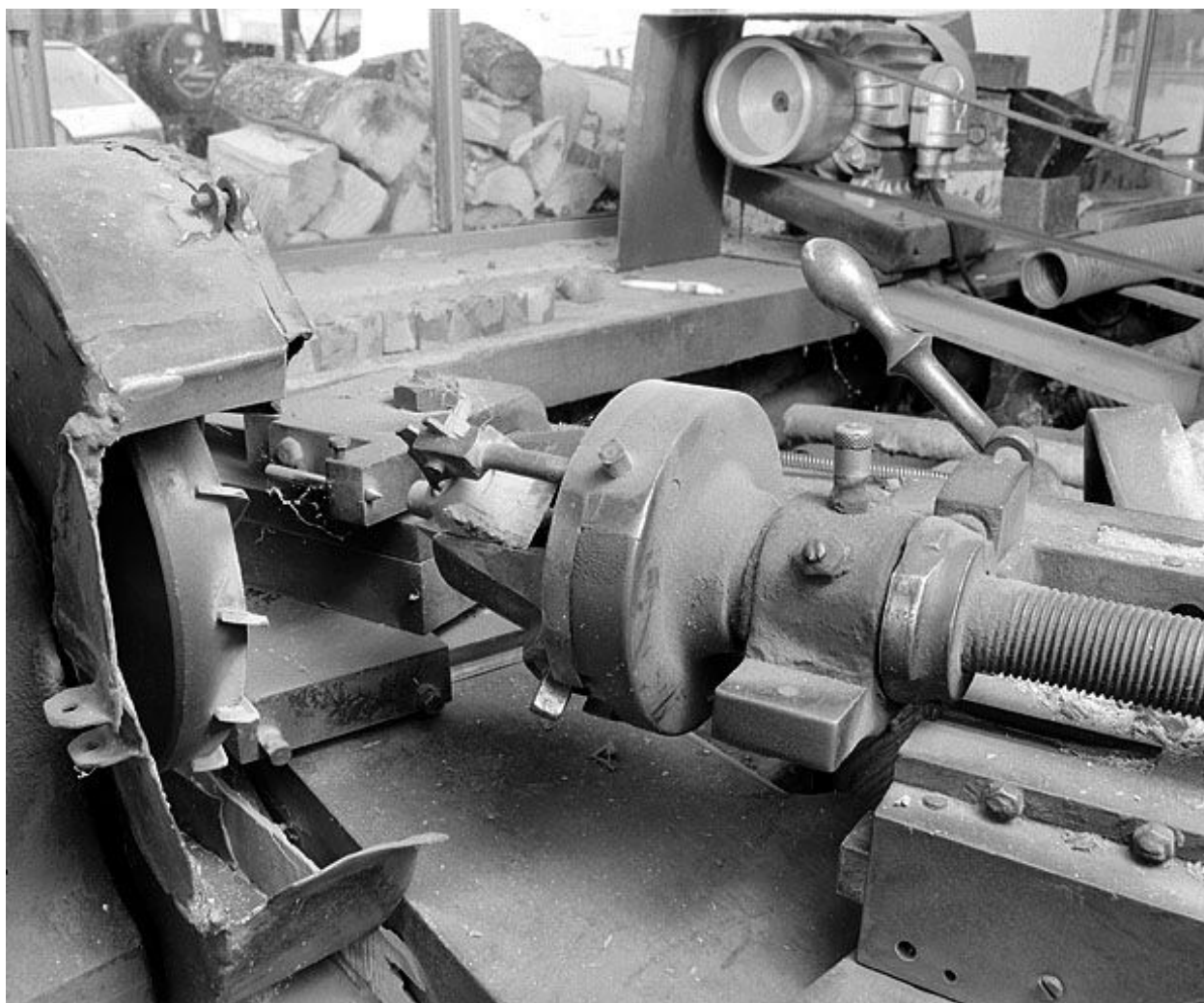
Mandrin gueule de loup et fraise verticale.
