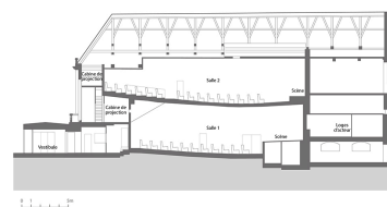
Coupe longitudinale. D'après une coupe fournie par les Services techniques de la Ville. Dess. Aline Thomas, Autr. auteur inconnu IVR26_20238900763NUDA
