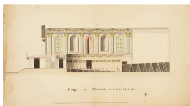
[Projet de salle de réunion et de spectacle dans l'église des capucins]. Coupe et élévation sur la ligne KK du plan. S.d. [entre 1792 et 1795]. Phot. Pierre-Marie Barbe-Richaud, Autr. Jacques Nicolas Caristie IVR26_20238900496NUC2A
