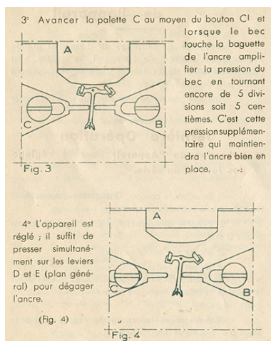
"Microchapp". Réglage [extrait d'un mode d'emploi, p. 5], fin des années 1940. IVR43_20182500471NUC4A
