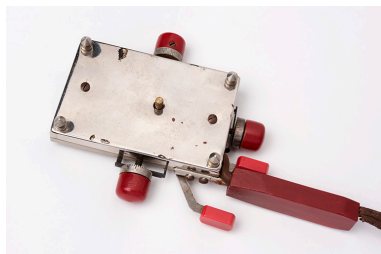
Microchapp d'origine : face inférieure. L'extrémité du tasseau en laiton portant le coussinet en rubis est visible au centre. Phot. Sonia Dourlot IVR43_20182500613NUC4A
