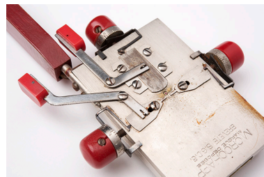
Microchapp d'origine, face supérieure : vue rapprochée. Le coussinet en rubis destiné à supporter le pivot de l'ancre est visible au centre, entre les deux palettes mobiles. Phot. Sonia Dourlot IVR43_20182500615NUC4A
