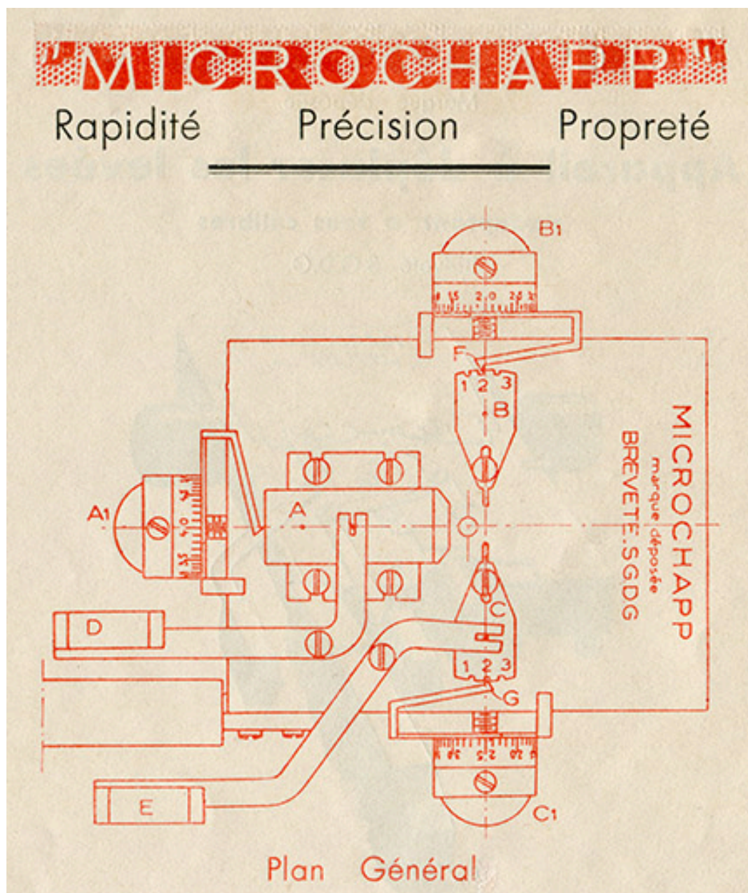
"Microchapp". Plan général [extrait d'un mode d'emploi, p. 2], fin des années 1940.
