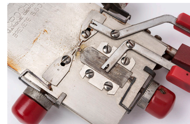
Microchapp d'origine, face supérieure : vue rapprochée (dans l'autre sens). Le coussinet en rubis destiné à supporter le pivot de l'ancre est visible entre les deux palettes mobiles. Phot. Sonia Dourlot IVR43_20182500614NUC4A
