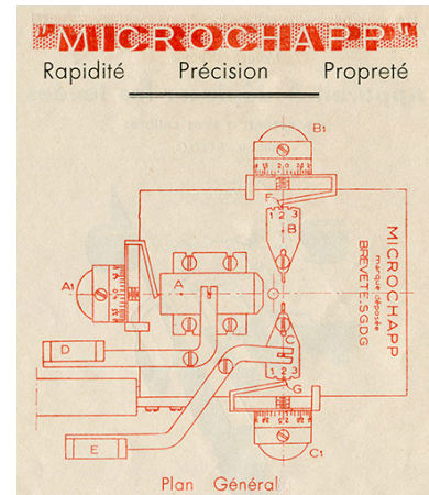
"Microchapp". Plan général [extrait d'un mode d'emploi, p. 2], fin des années 1940. IVR43_20182500470NUC4A
