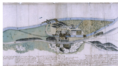
Plan de l'usine métallurgique de Moulin-Martin à Rigney : détail de la forge d'affinerie, 1647. Phot. Yves Sancey IVR43_19922500179XA
