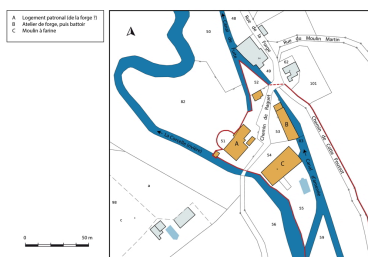
Plan-masse et de situation. Extrait du plan cadastral, 2019. Dess. Bertrand Turina IVR43_20192501042NUDA
