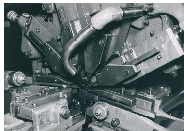
[6 burins Cardur montés sur une décolleteuse], 1978. IVR43_20162500134NUC2A
