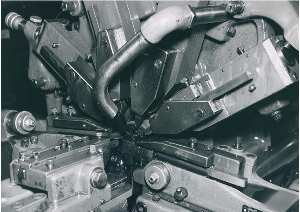
[6 burins Cardur montés sur une décolleteuse], 1978.
