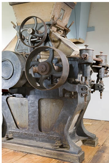
Appareil à cylindres Goulut-Borne. Détail. Phot. Jérôme Mongreville IVR43_20097000512NUC2A
