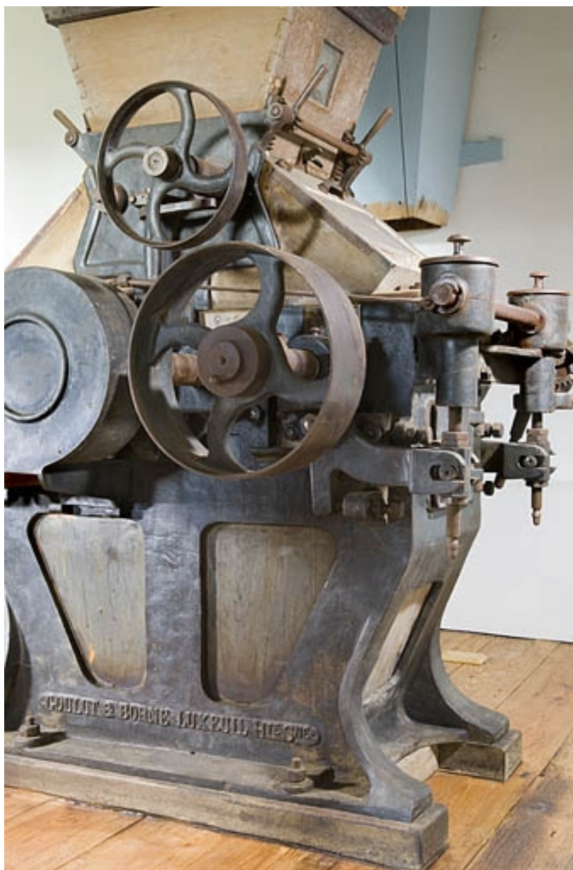
Appareil à cylindres Goulut-Borne. Détail.
