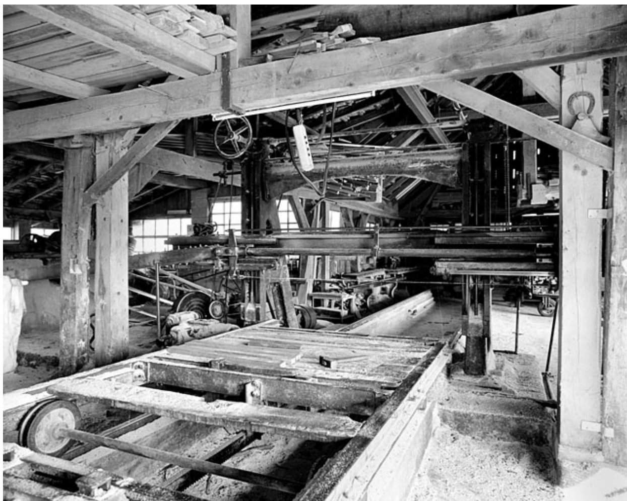
Châssis de scie horizontale monolame.
