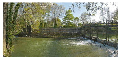
Barrage et vanne. Phot. Thierry Kuntz IVR26_20112102812NUC4A
