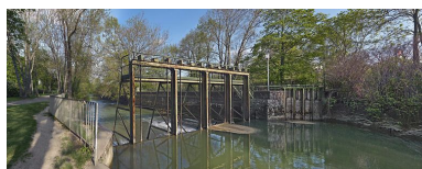
Barrage sur l'Ouche : la retenue d'eau en amont. Phot. Thierry Kuntz IVR26_20112102811NUC4A
