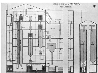
Coupe de la malterie. Phot. Raphaël Favereaux, Autr. IVR43_20122501330NUC2A
