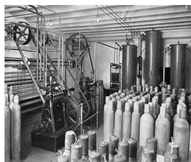
Récupération d'acide carbonique. Phot. Raphaël Favereaux, Autr. IVR43_20122501350NUC2A
