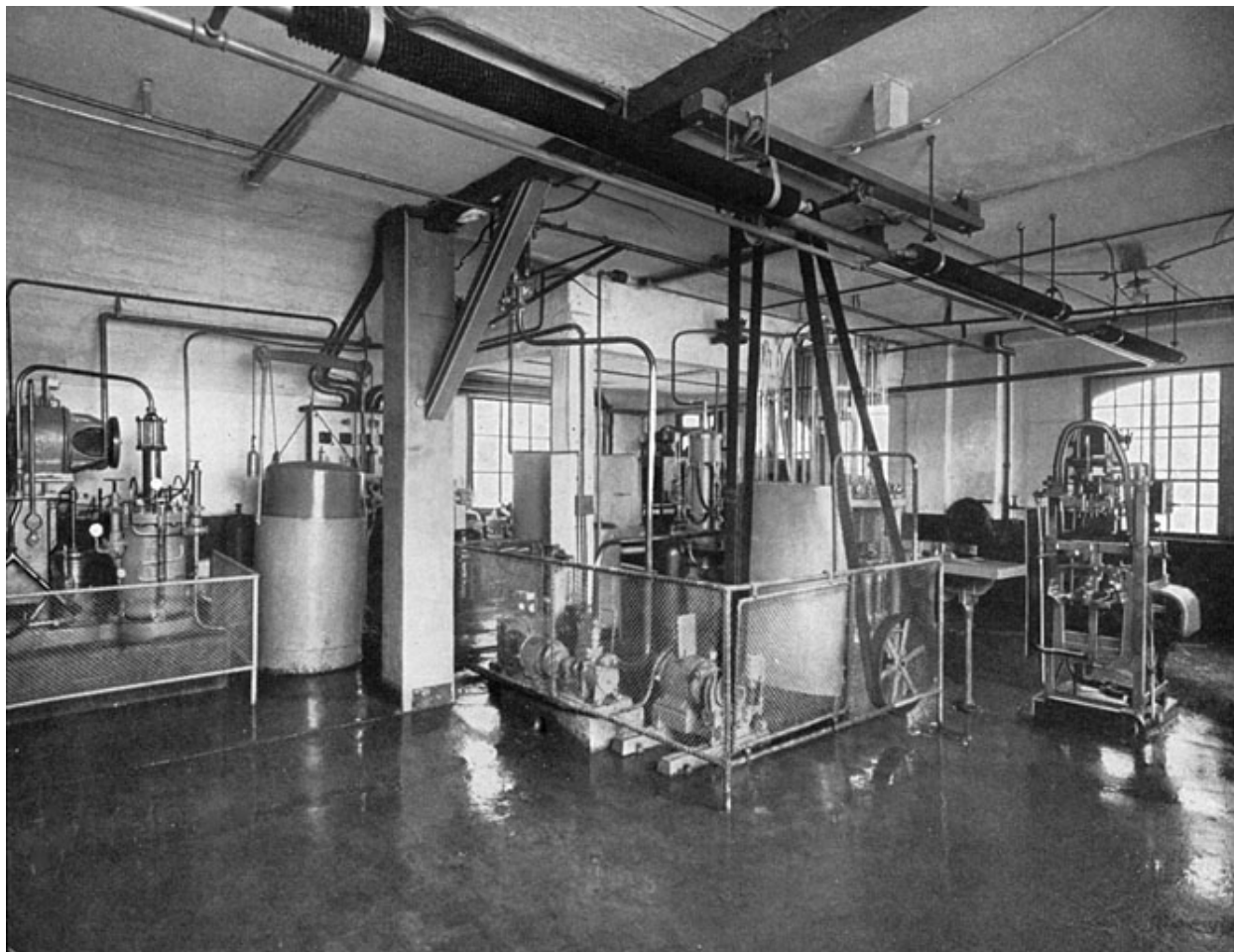
Fabrication des limonades (groupe de saturateur).
