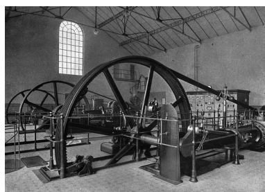
Salle des machines. Phot. Raphaël Favereaux, Autr. IVR43_20122501338NUC2A
