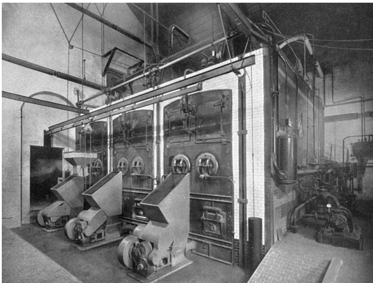
Générateurs (chaudière à charbon).
