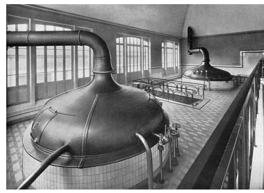
Chaudières à houblonner. Phot. Raphaël Favereaux, Autr. IVR43_20122501325NUC2A
