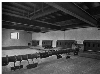
Touraille. Plateforme inférieure. Phot. Raphaël Favereaux, Autr. IVR43_20122501349NUC2A
