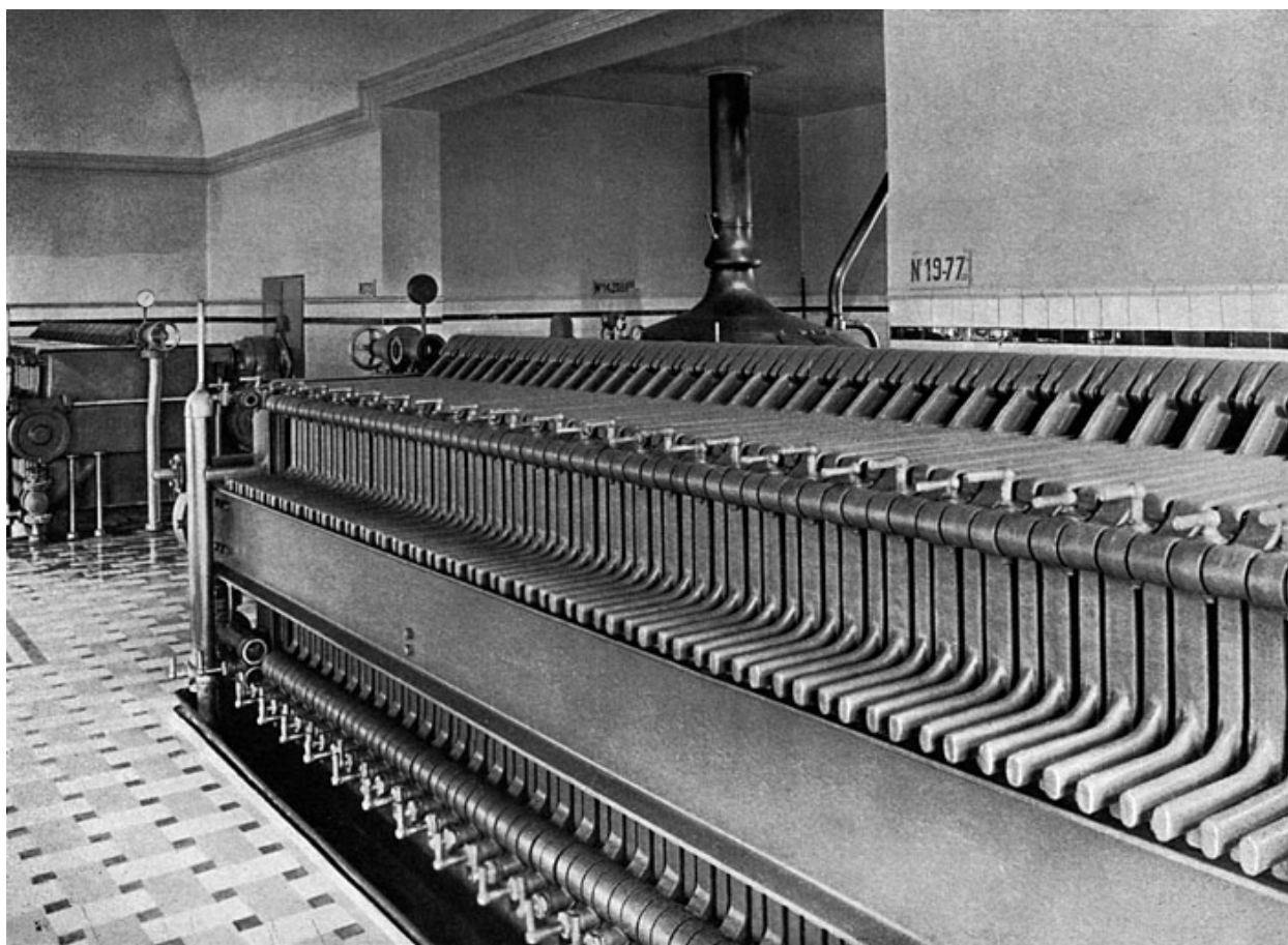
Filtre à moût.
