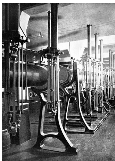
Soutireuses isobarométriques. Phot. Raphaël Favereaux, Autr. IVR43_20122501344NUC2A
