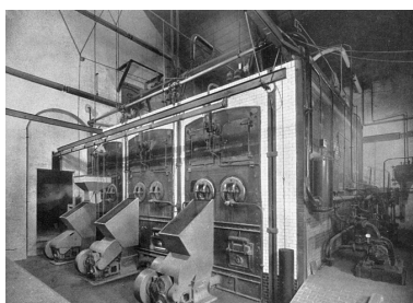
Générateurs (chaudière à charbon). Phot. Raphaël Favereaux, Autr. IVR43_20122501339NUC2A
