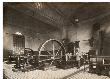
Salle des machines. Phot. Jérôme Mongreville IVR43_20132500482NUC4A
