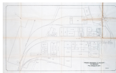
Grandes Brasseries et Malteries de Sochaux. Plan général de l'usine, 1927. Phot. Jérôme Mongreville IVR43_20132500511NUC4A
