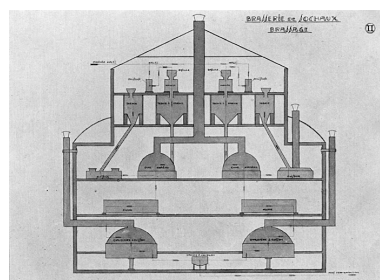
Coupe de la salle de brassage. Phot. Raphaël Favereaux, Autr. IVR43_20122501331NUC2A
