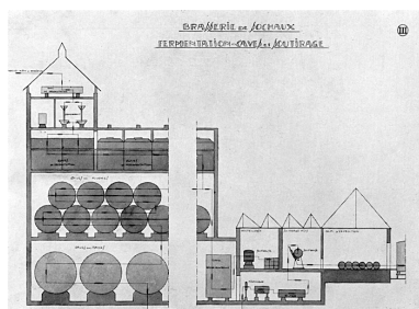
Coupe des caves de fermentation et du soutirage. Phot. Raphaël Favereaux, Autr. IVR43_20122501332NUC2A
