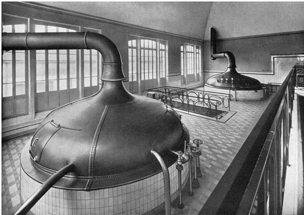
Chaudières à houblonner.
