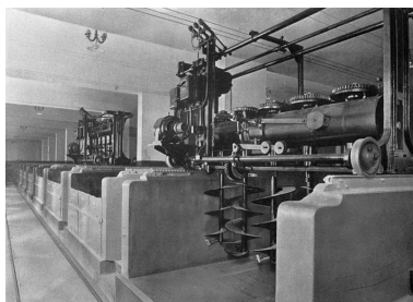
Germoirs et retourneurs automatiques. Phot. Raphaël Favereaux, Autr. IVR43_20122501336NUC2A
