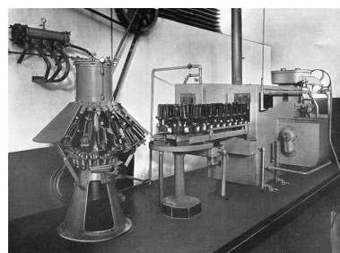
Embouteillage de la bière. Phot. Raphaël Favereaux, Autr. IVR43_20122501334NUC2A
