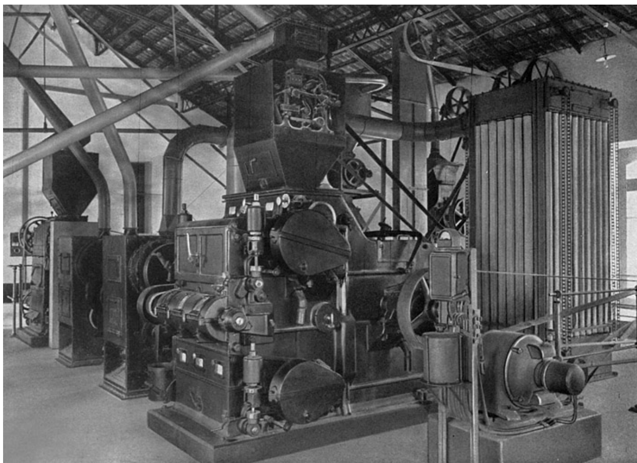
Moulins concasseurs.
