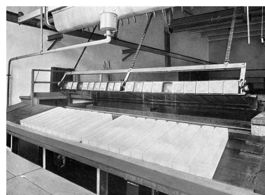
Générateur à glace. Phot. Raphaël Favereaux IVR43_20122501346NUC2A
