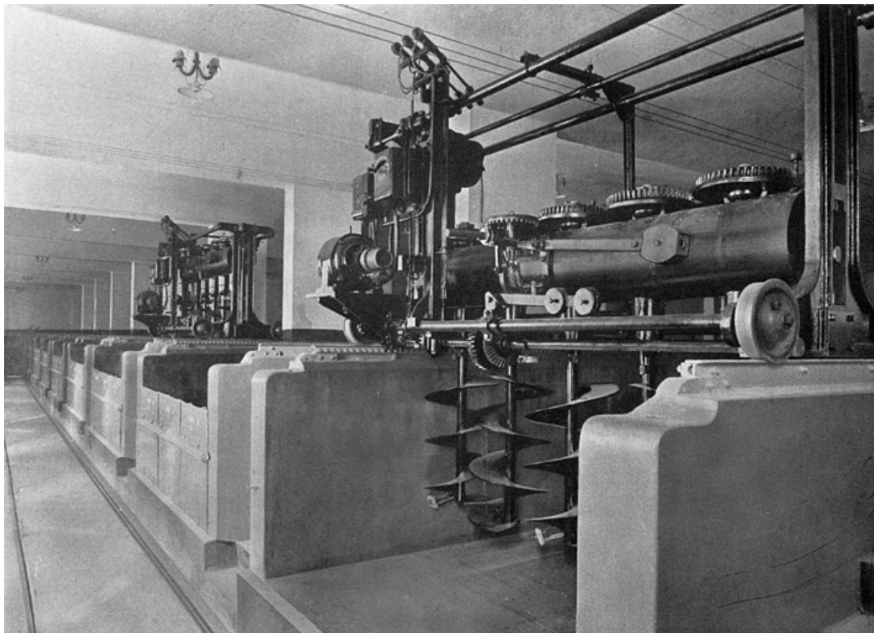
Germoirs et retourneurs automatiques.
