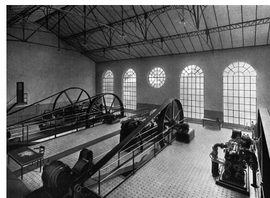
Salle des machines. Phot. Raphaël Favereaux, Autr. IVR43_20122501337NUC2A
