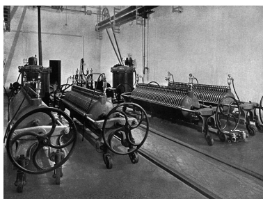
Salle des filtres. Phot. Raphaël Favereaux, Autr. IVR43_20122501327NUC2A
