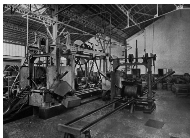
Lavage des fûts. Phot. Raphaël Favereaux, Autr. IVR43_20122501326NUC2A
