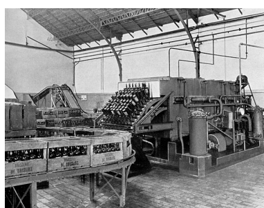
Laveuse. Phot. Raphaël Favereaux, Autr. IVR43_20122501341NUC2A
