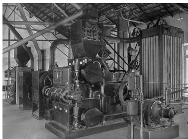
Moulins concasseurs. Phot. Raphaël Favereaux, Autr. IVR43_20122501321NUC2A
