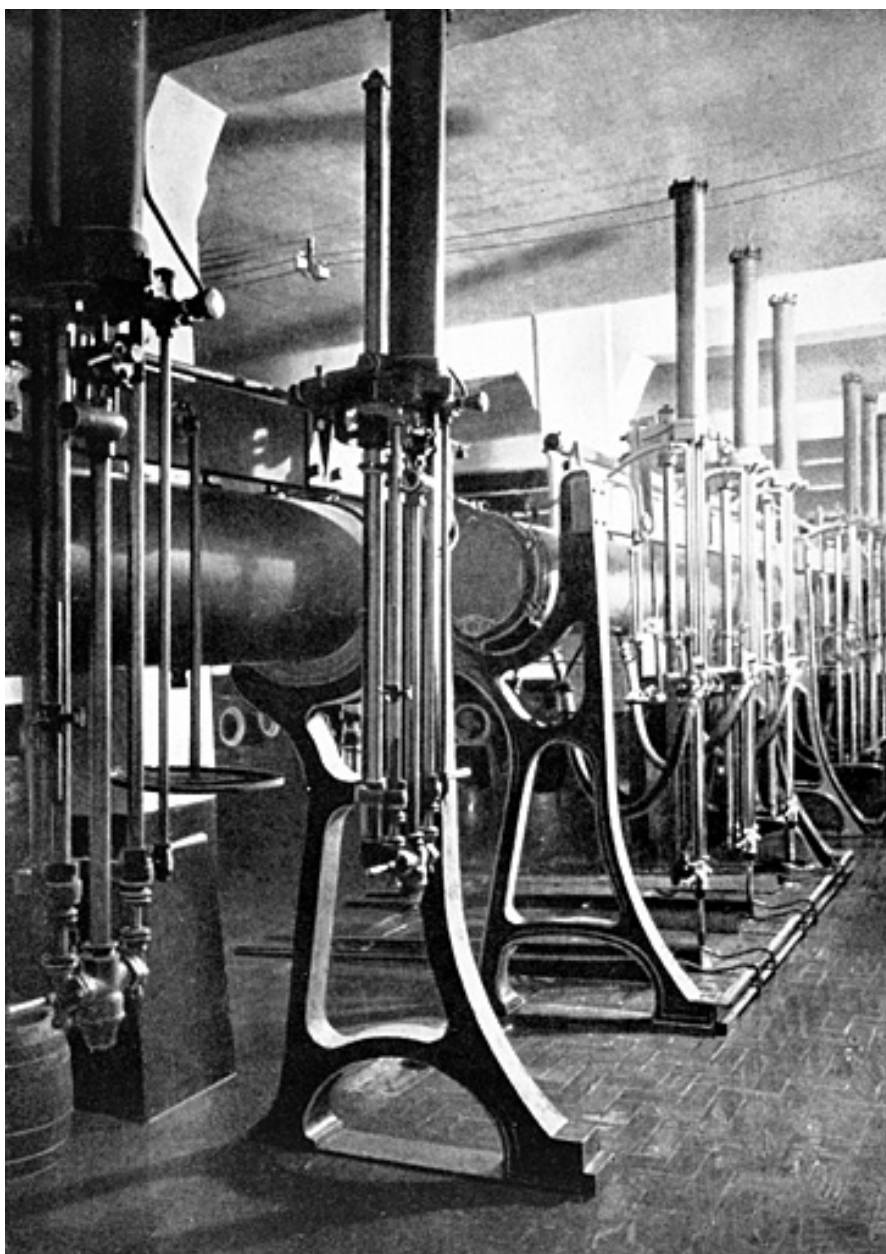
Soutireuses isobarométriques.
