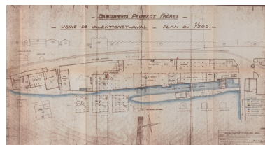
Ets Peugeot Frères. Usine de Valentigney-aval [partie nord]. Plan, échelle 1/500, s.n., 1962. Autr. IVR43_20122501690NUC2A
