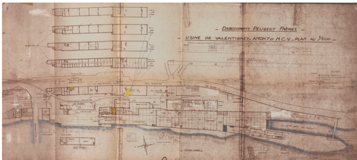
Ets Peugeot Frères. Usine de Valentigney-amont [partie sud]. Plan, échelle 1/500, s.n., 1962.
