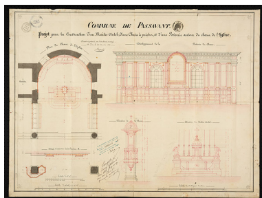
Projet de construction d'un maître-autel pour l'église Notre-Dame (1862). Phot. Sonia Dourlot, Autr. Pierre Mougenot IVR43_20167000049NUC4A
