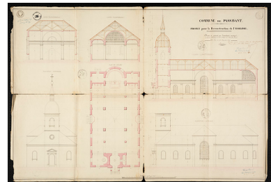
Projet pour la reconstruction de l'église. Phot. Sonia Dourlot, Autr. Pierre Mougenot IVR43_20167000046NUC4A
