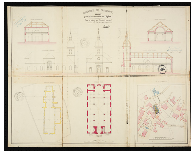
Plan pour la reconstruction de l'église. Phot. Sonia Dourlot, Autr. Pierre Mougenot IVR43_20167000047NUC4A
