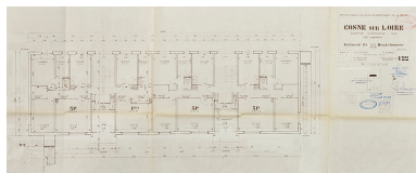
Opération de 226 logements : bâtiment B1, plan du rez- de-chaussée ; J. Louria, F. Sonnet, mars 1970. (Archives municipales Cosne-Cours- sur-Loire, 200 W 117 - PC 1015) Phot. Thierry Kuntz, Autr. Jean Louria, Autr. F. Sonnet (architecte d'opération) IVR26_20145800200NUC4A
