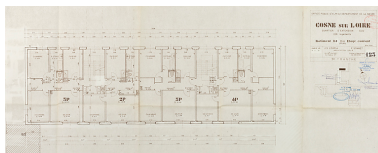
Opération de 226 logements : bâtiment B1, plan d'étage courant ; J. Louria, F. Sonnet, mars 1970. (Archives municipales Cosne-Cours- sur-Loire, 200 W 117 - PC 1015) Phot. Thierry Kuntz, Autr. Jean Louria, Autr. F. Sonnet (architecte d'opération) IVR26_20145800201NUC4A
