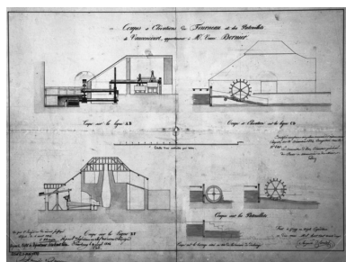
Coupes et élévations du fourneau et des patouilletts de Vauconcourt, appartenant à Mme veuve Dornier. Phot. Yves Sancey, Autr. Auguste Sirodot IVR43_19877000085X
