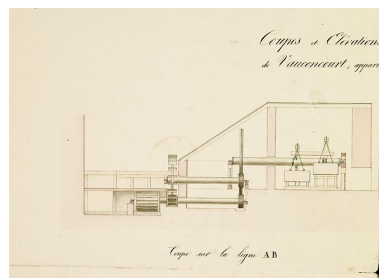
Coupes et élévations du fourneau et des patouilletts de Vauconcourt [coupe transversale]. Phot. Jérôme Mongreville, Autr. Auguste Sirodot IVR43_20097000029NUC2A
