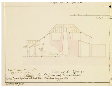
Coupes et élévations du fourneau et des patouilletts de Vauconcourt [coupe du haut fourneau]. Phot. Jérôme Mongreville, Autr. Auguste Sirodot IVR43_20097000030NUC2A
