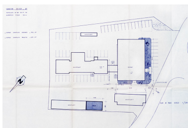
S.B.B.M. 25 – Damprichard. Plan de masse, 27 août 1972. Phot. Jérôme Mongreville, Autr. Pierre Joly IVR43_20132500570NUC4A
