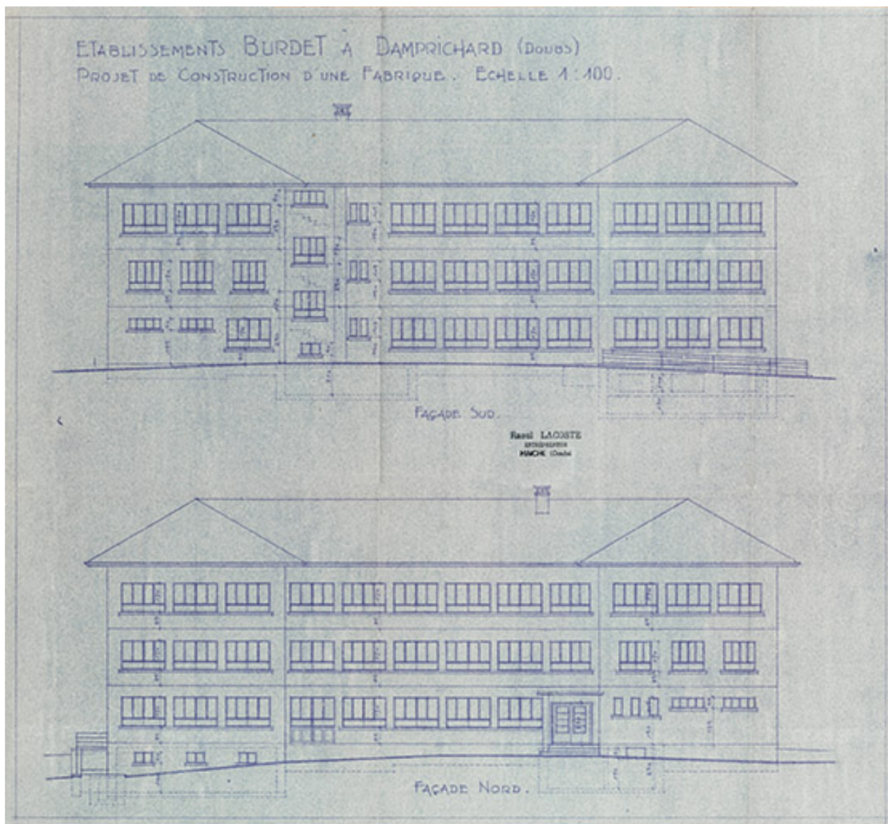
Établissements Burdet à Damprichard (Doubs). Projet de construction d'une fabrique [élévations sud et nord], [1951].
