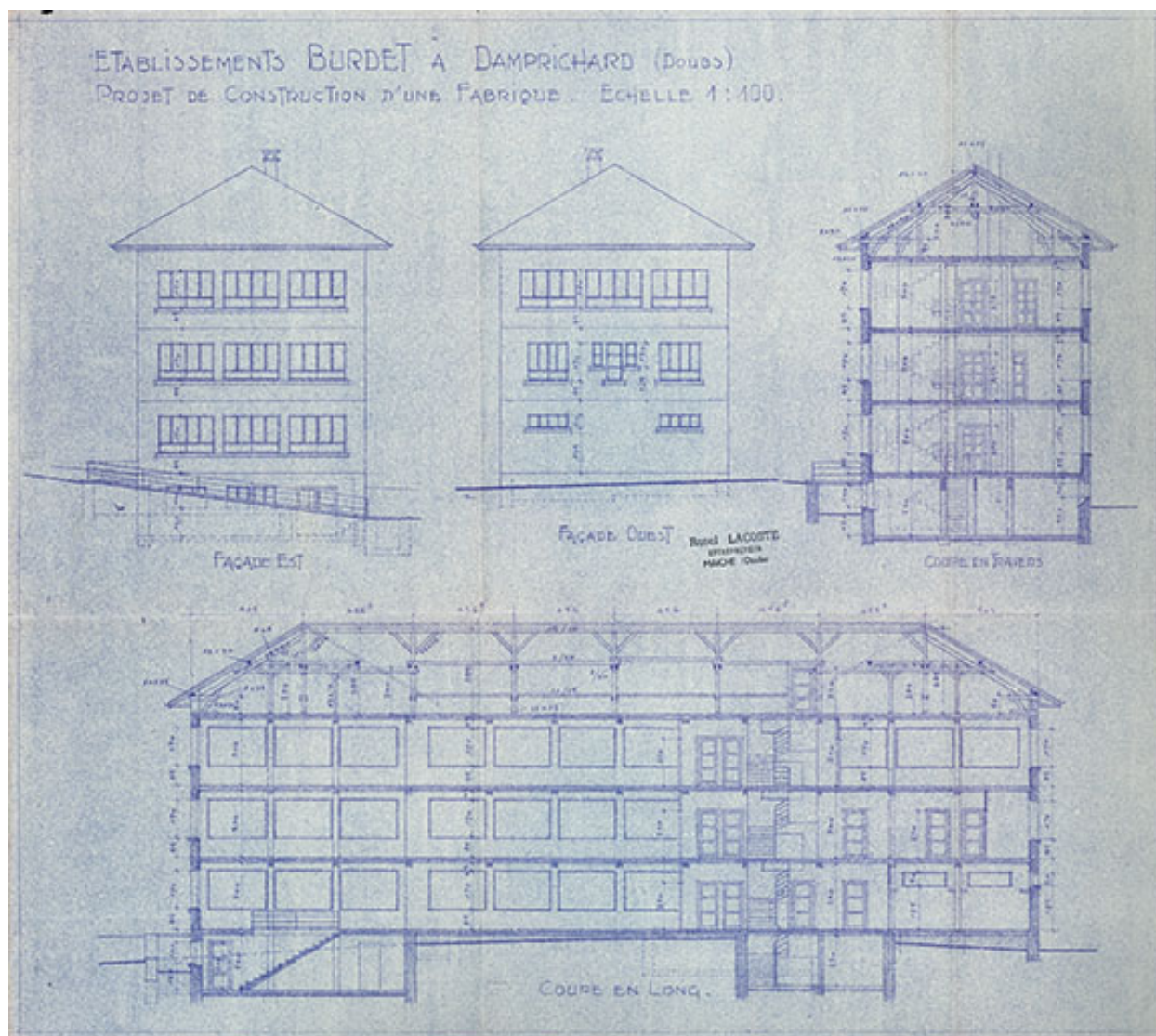
Établissements Burdet à Damprichard (Doubs). Projet de construction d'une fabrique [coupes et élévations est et ouest], [1951].
