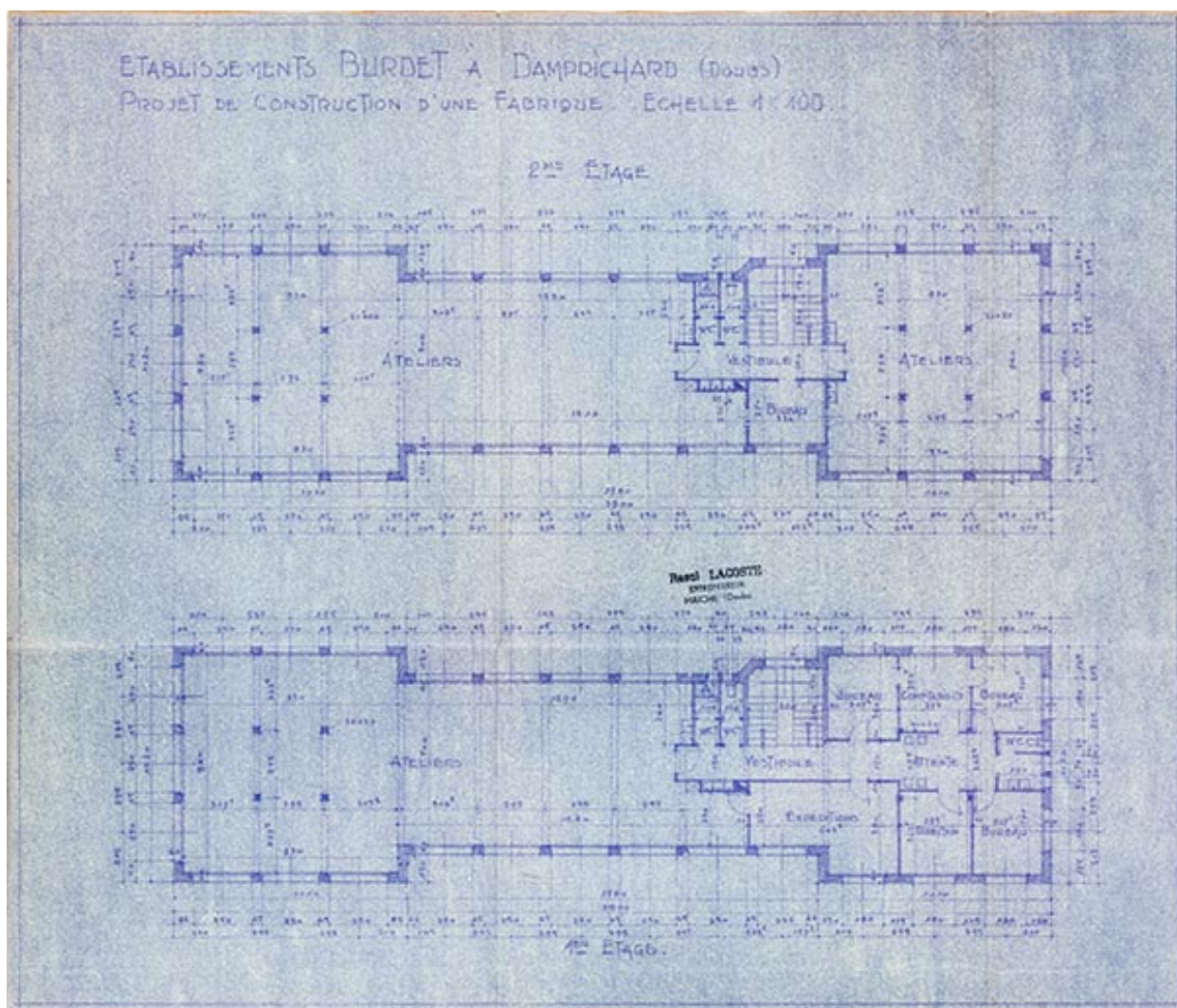
Établissements Burdet à Damprichard (Doubs). Projet de construction d'une fabrique [plan du 1er et du 2e étage], [1951].
