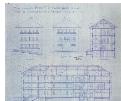
Établissements Burdet à Damprichard (Doubs). Projet de construction d'une fabrique [coupes et élévations est et ouest], [1951].
