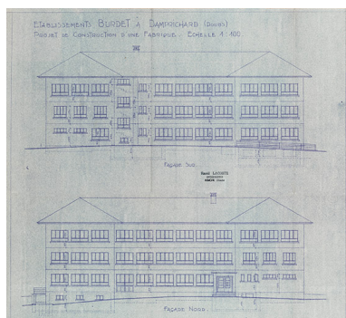
Établissements Burdet à Damprichard (Doubs). Projet de construction d'une fabrique [élévations sud et nord], [1951]. Phot. Jérôme Mongreville, Autr. Raoul Lacoste IVR43_20132500585NUC4A
