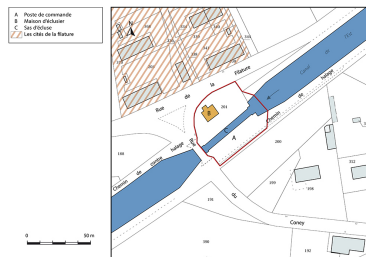
Plan de masse et de situation. Dess. Mathias Papigny IVR43_20177000359NUDA
