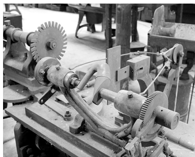
Détail de la partie où se fixe la pièce à copier. Phot. Yves Sancey IVR43_20022500871X
