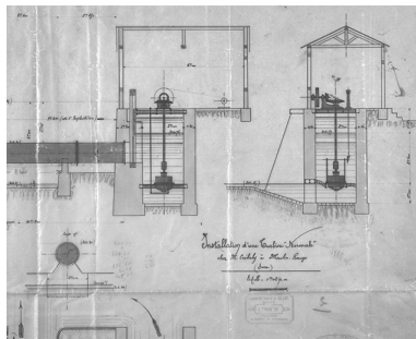
Installation d'une Turbine " Normale " chez M. Crébely à Moulin-Rouge (Jura). Phot. Yves Sancey, Autr. Ets Laurent Frères et Collot IVR43_19893901169X
