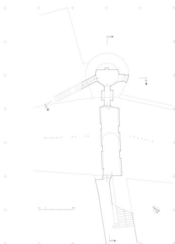
Tour Notre-Dame. Plan du niveau inférieur. Dess. Alain Morelière IVR26_20122100098A2YY
