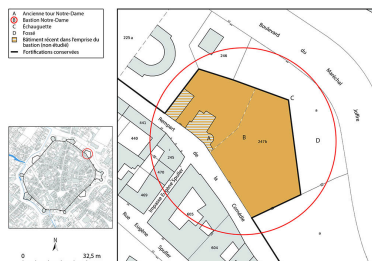
Plan-masse et de situation. Extrait du plan cadastral, 2024, 1/650. Dess. Aline Thomas IVR26_20242100041NUDA
