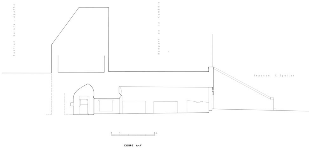
Tour Notre-Dame. Coupe A-A'.
