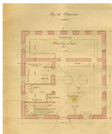
Construction d'un chalet-modèle. Plan du rez-de-chaussée, 1905. IVR43_20192500090NUC4A
