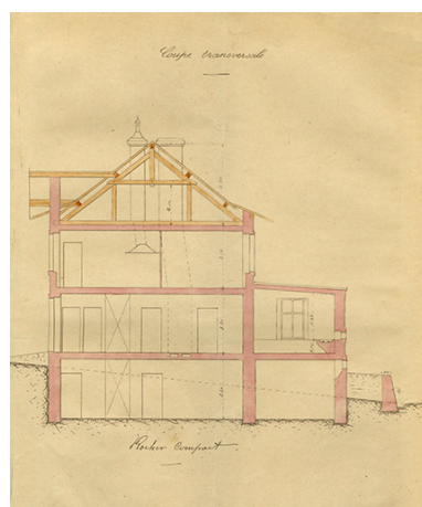
Construction d'un chalet-modèle. Coupe transversale, 1905. IVR43_20192500093NUC4A
