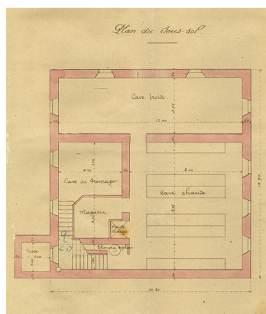
Construction d'un chalet-modèle. Plan du sous-sol, 1905. IVR43_20192500091NUC4A
