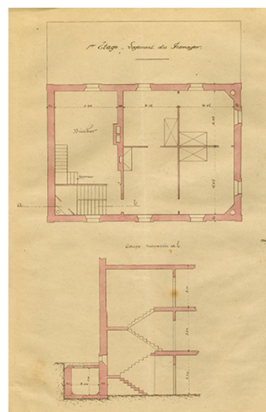
Construction d'un chalet-modèle. Plan du 1er étage, 1905. IVR43_20192500092NUC4A
