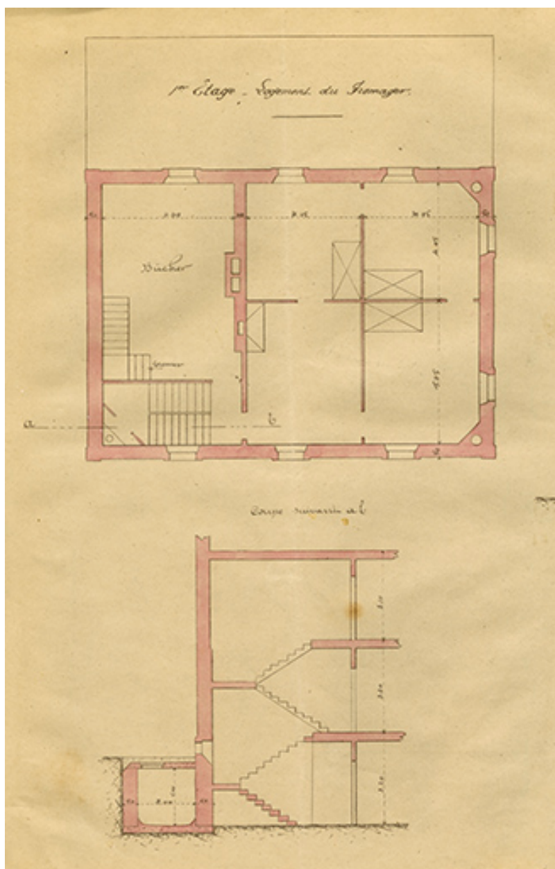
Construction d'un chalet-modèle. Plan du 1er étage, 1905.
