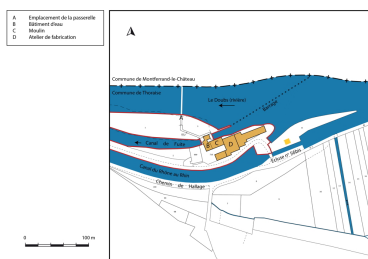
Plan-masse et de situation. Extrait du plan cadastral, 2019. Dess. Bertrand Turina IVR43_20192501058NUDA
