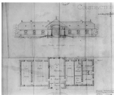
Commune de Desnes. Construction d'un Chalet. [Détail : façade principale et plan au rez de chaussée]. Phot. Jérôme Mongreville, Phot. Jules Pelletier IVR43_19963900213X
