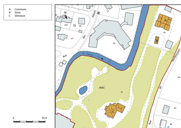
Plan-masse et de situation. Dess. Mathias Papigny IVR43_20132502631NUDA
