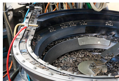
Atelier d'assemblage : détail du bol d'alimentation.
