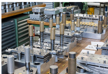
Atelier de fabrication de l'outillage : étau progressives (ou outils à suivre). Phot. Sonia Dourlot IVR43_20162501225NUC4A
