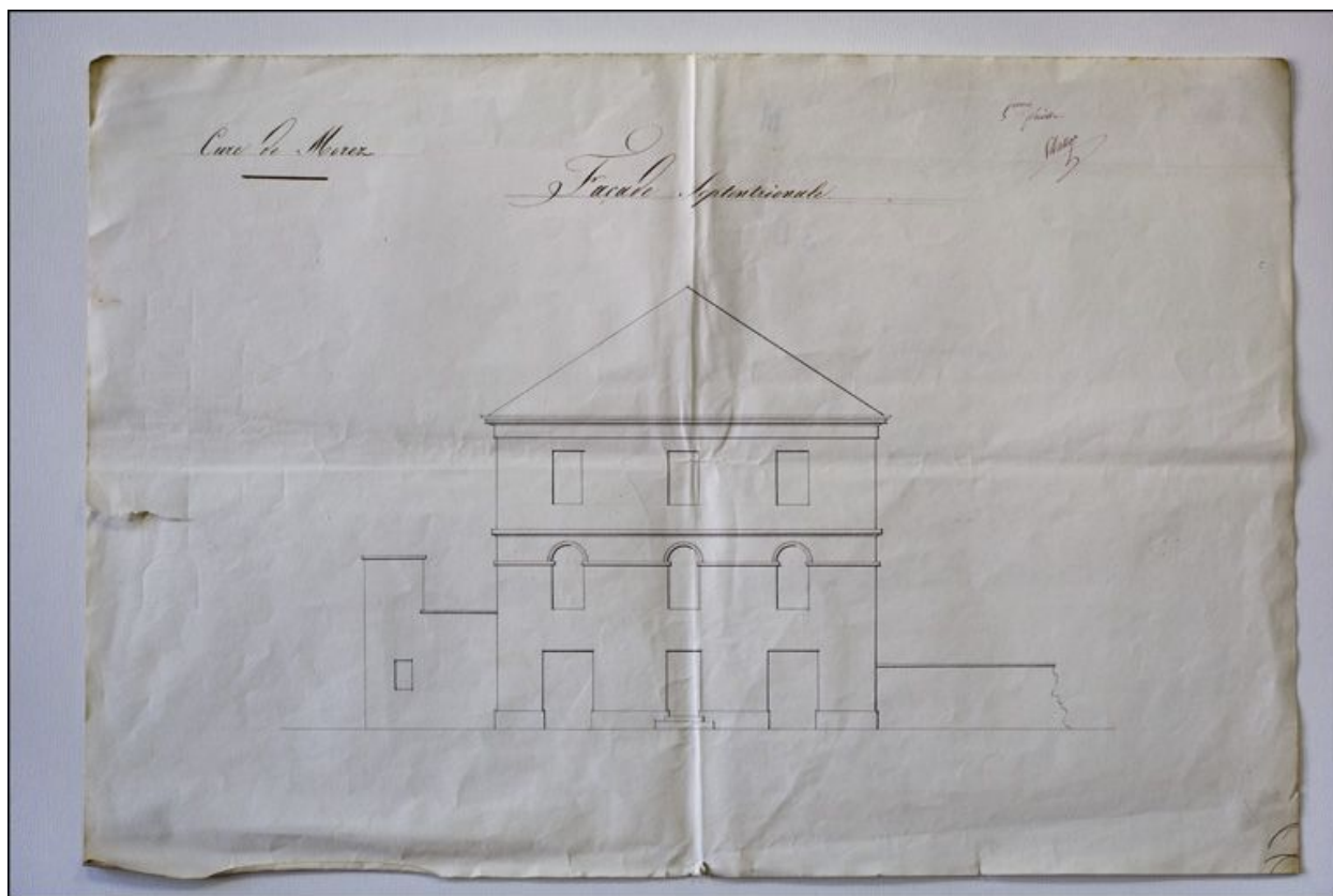
Cure de Morez. 5e feuille. Façade septentrionale, 1836. Dessin (plume), [mars] 1836, sans échelle [1:100].
