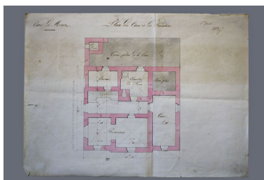
Cure de Morez. 1ère feuille. Plan des caves et des fondations, 1836. Dessin (plume, lavis), [mars] 1836, sans échelle [1:100]. Phot. Yves Sancey, Autr. Claude-Marie (architecte d'arrondissement) Dalloz IVR43_20103900037NUC2A
