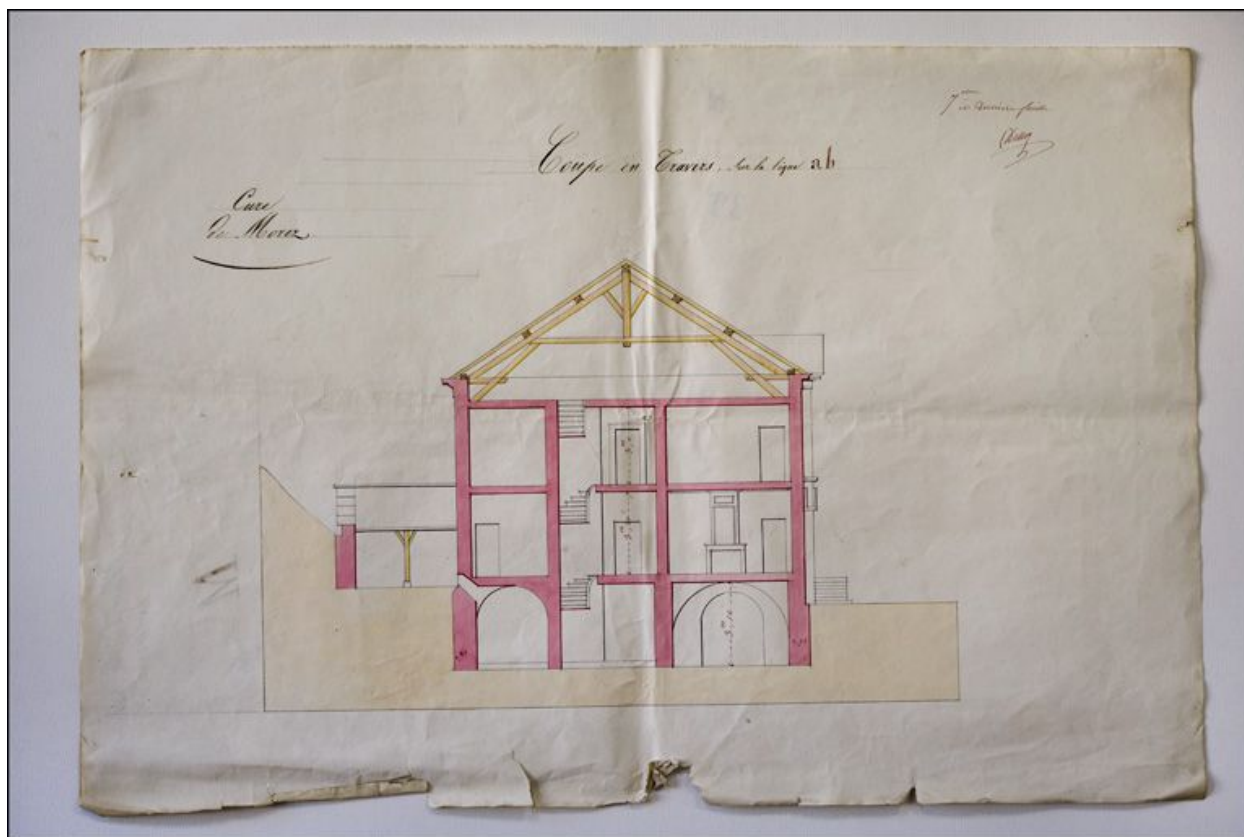
Cure de Morez. 7e et dernière feuille. Coupe en travers sur la ligne ab, 1836. Dessin (plume, lavis), [mars] 1836, sans échelle [1:100].
