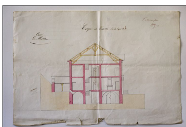
Cure de Morez. 7e et dernière feuille. Coupe en travers sur la ligne ab, 1836. Dessin (plume, lavis), [mars] 1836, sans échelle [1:100]. Phot. Yves Sancey, Phot. Claude-Marie Dalloz IVR43_20103900041NUC2A
