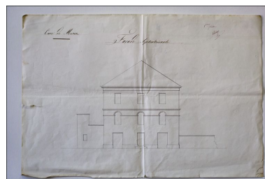
Cure de Morez. 5e feuille. Façade septentrionale, 1836. Dessin (plume), [mars] 1836, sans échelle [1:100]. Phot. Yves Sancey, Phot. Claude-Marie Dalloz IVR43_20103900040NUC2A
