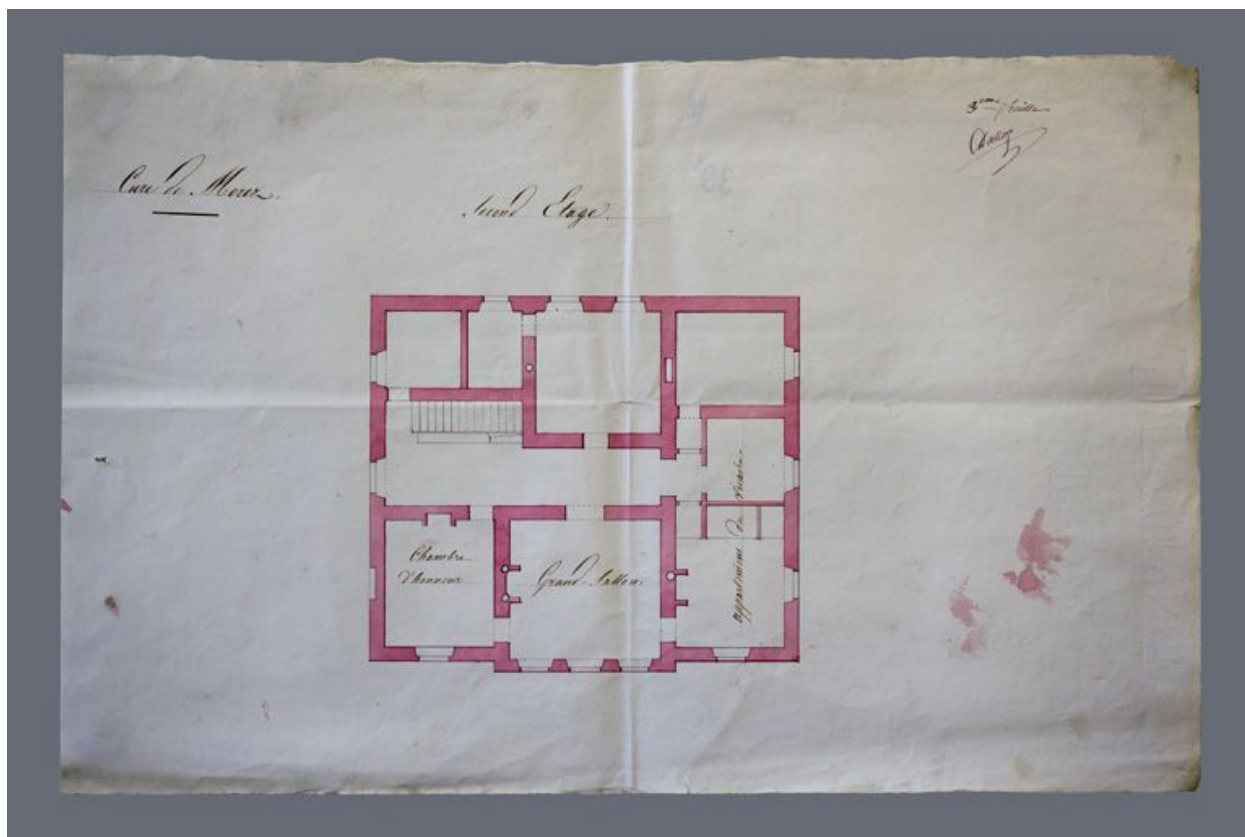
Cure de Morez. 3e feuille. Second étage, 1836. Dessin (plume, lavis), [mars] 1836, sans échelle [1:100].
