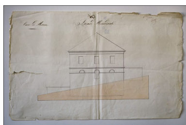
Cure de Morez. 6e feuille. Façade méridionale, 1836. Dessin (plume, lavis), [mars] 1836, sans échelle [1:100]. Phot. Yves Sancey, Autr. Claude-Marie (architecte d'arrondissement) Dalloz IVR43_20103900039NUC2A
