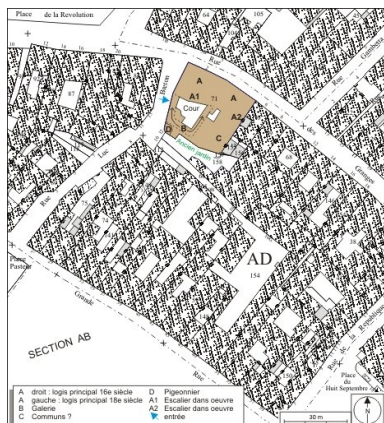
Plan masse et de situation. Extrait du plan cadastral, 1974, section AD. Dess. André Céréza IVR43_20102500054NUDA
