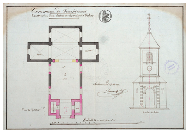
Projet de construction d'un clocher à l'église, plan des fondations (1843).
