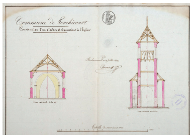
Projet de construction d'un clocher à l'église, coupe (1843).
