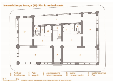
Plan du rez-de-chaussée, échelle 1/200, mise au net d'un relevé, s.d. [vers 1875].
